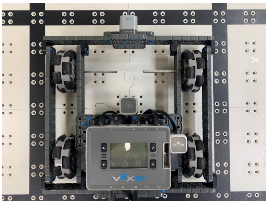
圖 11.雷射距離感測器研究車輛外觀
