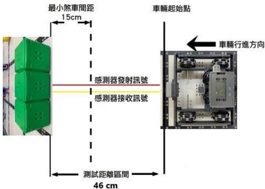
圖 14.場地規劃圖
