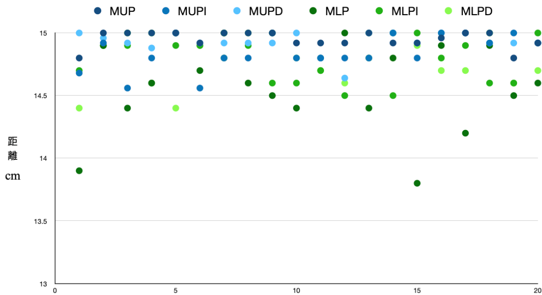
圖 21.移動障礙物之間距離數值分布圖
