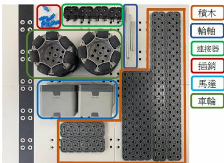
圖 7. 基本結構材料
