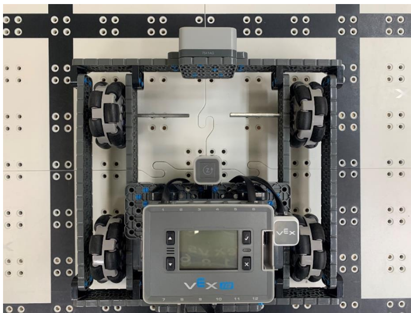
圖 10.超音波距離感測器研究車輛外觀
