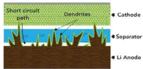
圖 1-3-4 鋰金屬樹枝狀結構造成短路示意圖 (圖片來源：CASE 報科學(國立台灣大學)-材料科技-鋰電池樹枝狀結晶的難題)
