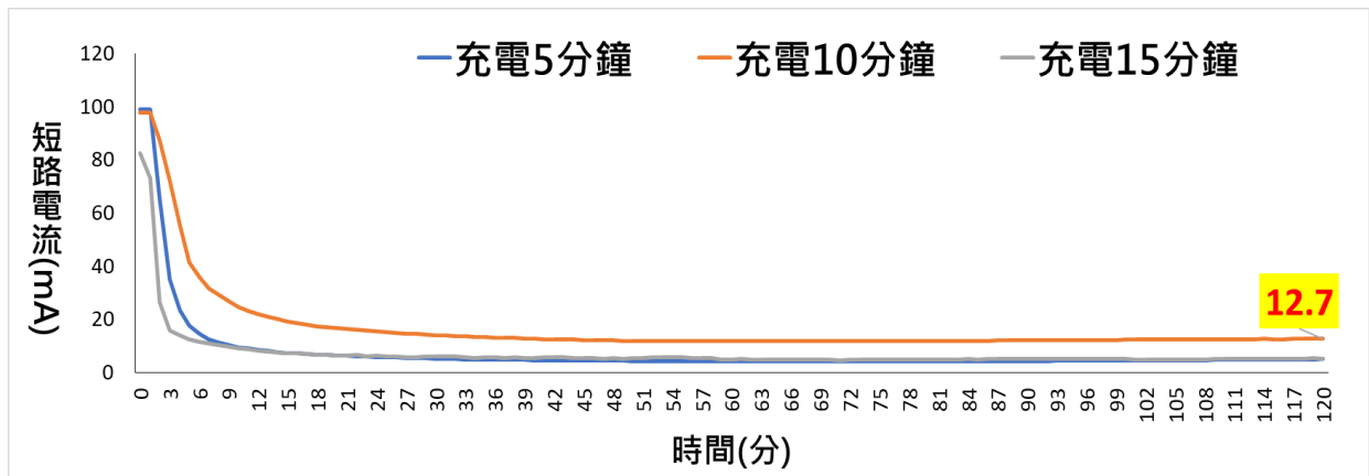
圖 3-3-8-4 自製電池在充電不同時間後，其 2 小時間的放電電流值
