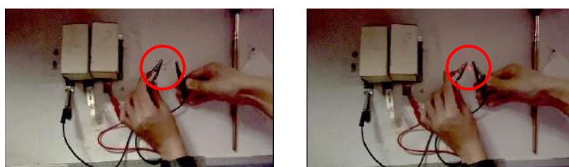
圖 3-3-8-2 將兩個電池分別充電 5 分鐘，串聯後成功點亮 LED 燈，並持續至少 190 天 (截至 113/10/24) (照片皆由第一作者拍攝)。
