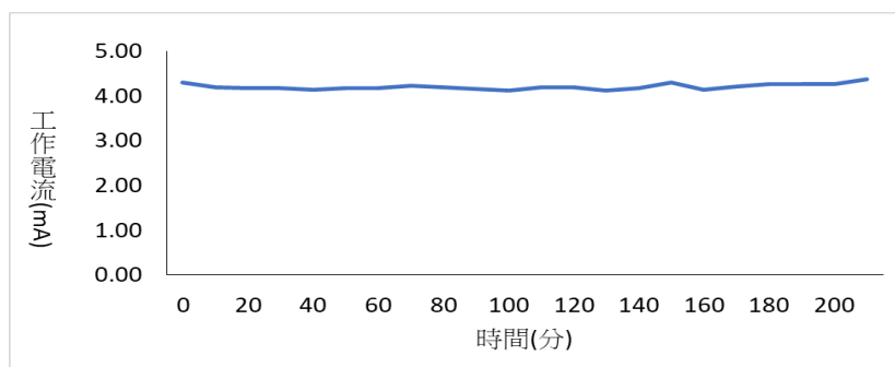
圖 3-3-8-6 自製電池在接上風扇後，其 3.5 小時的工作電流值
