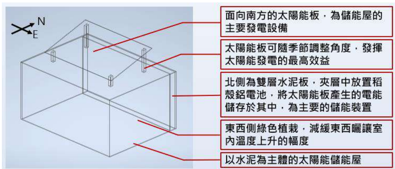
圖 3-3-9-3 太陽儲能屋初步的設計概念圖(兩位作者畫草圖，再由指導老師幫忙繪製)
