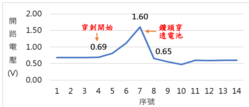
圖 3-3-8-10 穿刺實驗的開路電壓值
