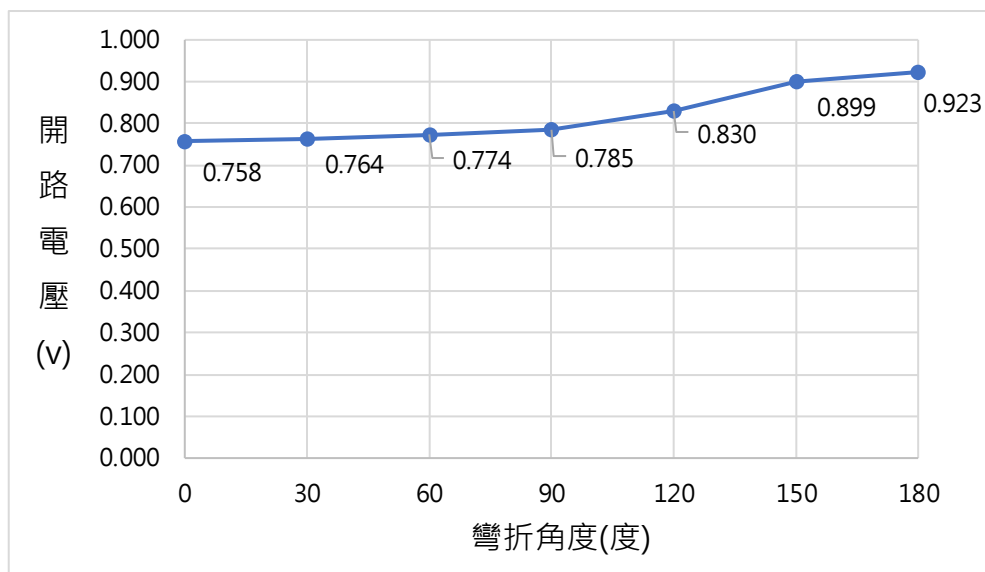
圖 3-3-8-8 彎折實驗的開路電壓值
