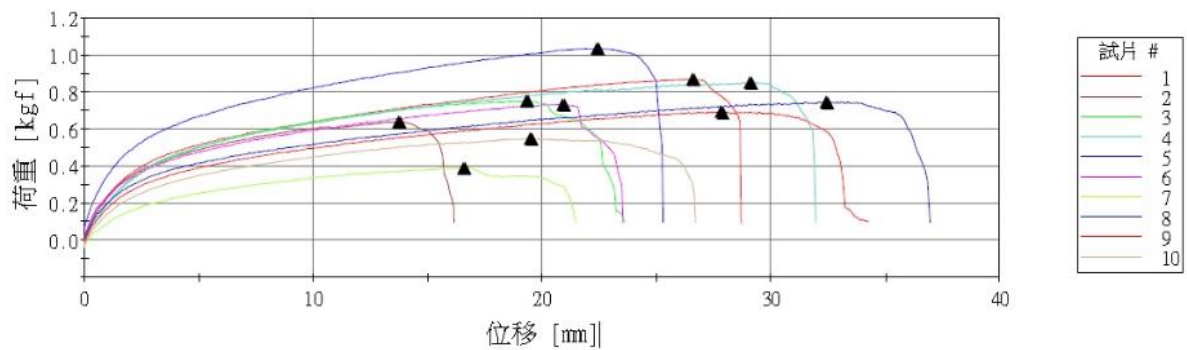
圖 9 拉伸強度實驗
