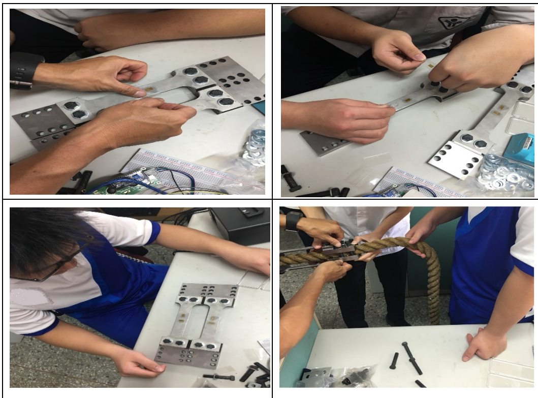
圖 17、黏貼應變規的過程
