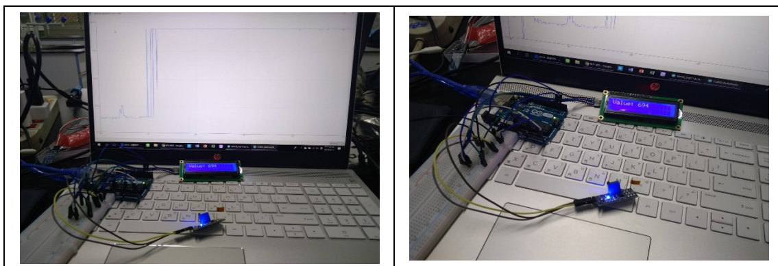
圖 12、使用 LCD 顯示出應變規的應變量量值
