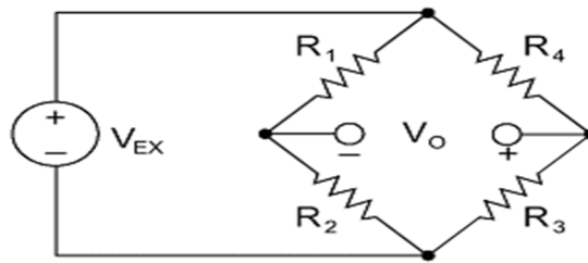
圖 5、Wheatstone 橋接電路使用應變規組態來偵測微小的電阻變化
