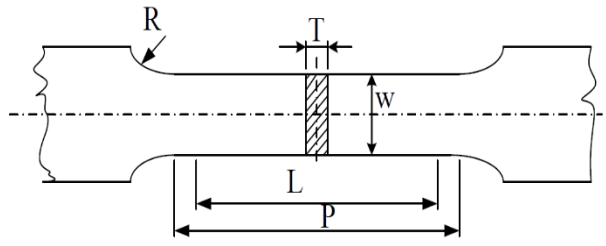
(b) 扁平形試樣
