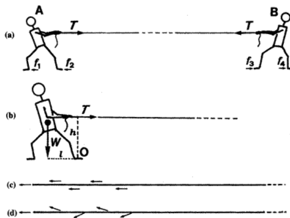
圖 7、拔河時張力 T 的示意圖
