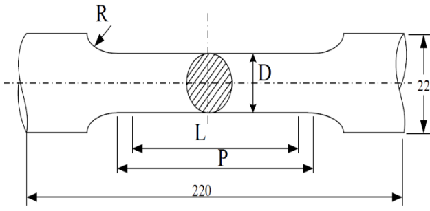
(a) 圓形試樣
