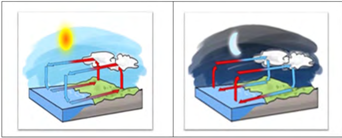
圖 35 海風、陸風示意圖
