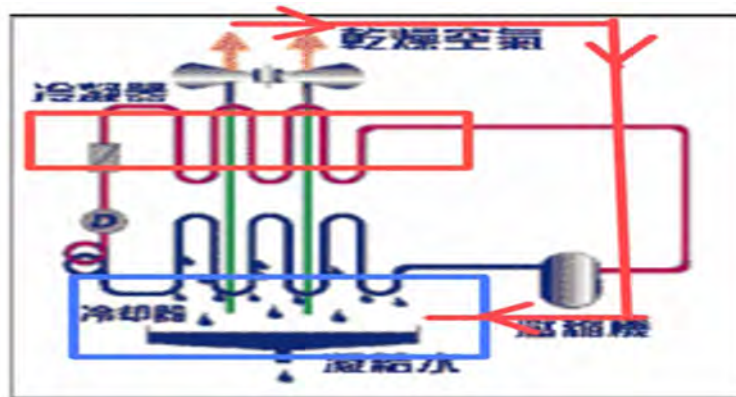
圖 37 水氣蒸散凝結示意圖(除溼機原理)
