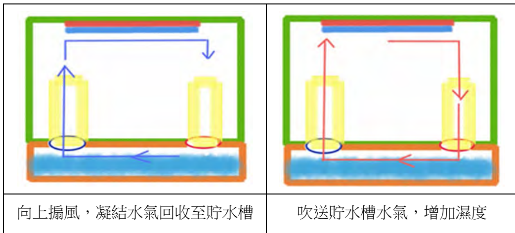
圖 36 自製植物箱貯水槽水氣流動示意圖
