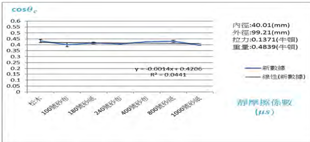
圖94實驗數據圖
