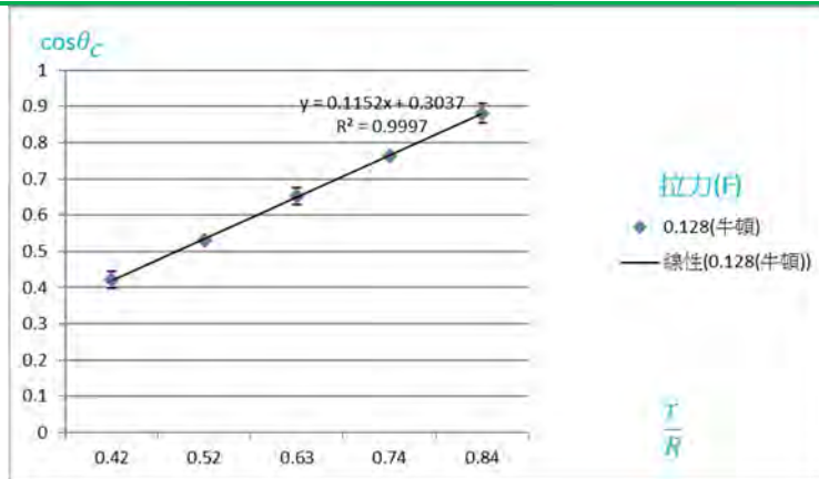
圖56 \cos \theta_c 與線軸內外徑比值之關係圖
