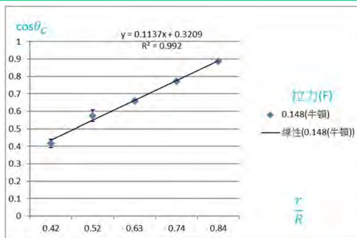
圖58 \cos \theta_c 與線軸內外徑比值之關係圖
