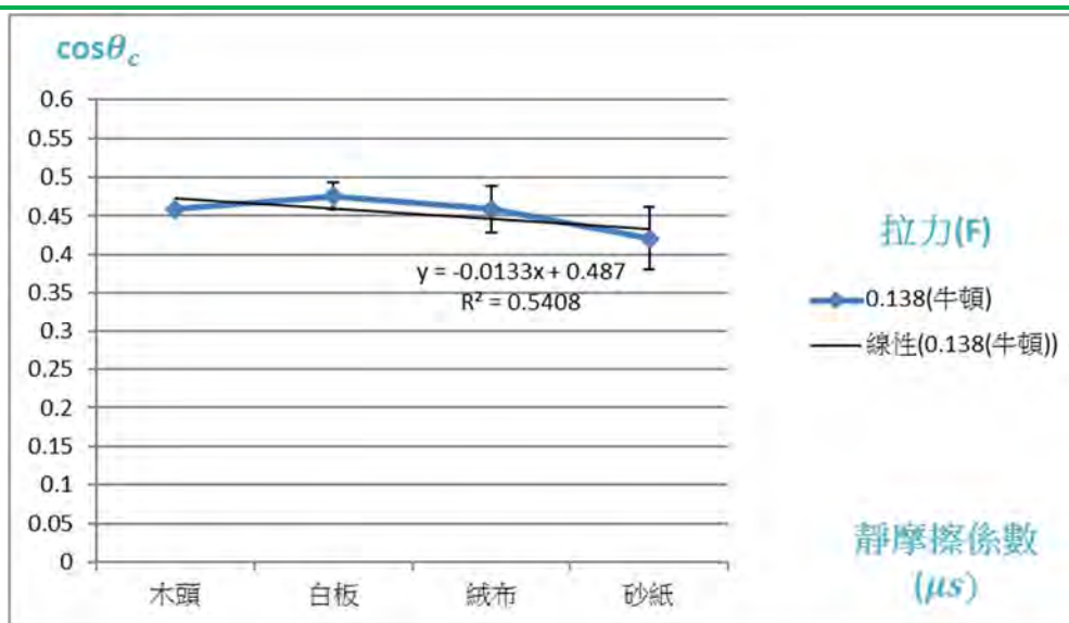
圖71 \cos \theta_c 與靜摩擦係數之關係圖
