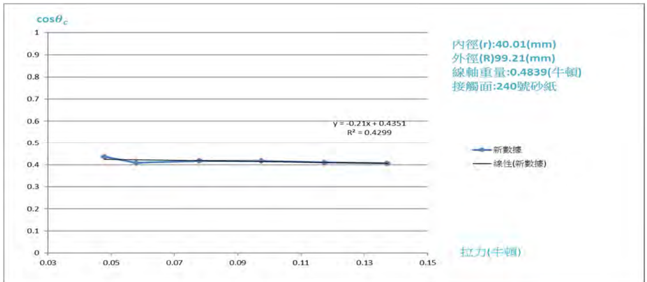
圖 91 實驗數據圖
