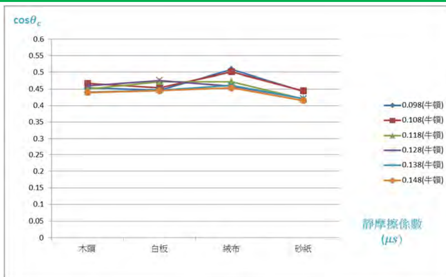
圖73 \cos \theta_c 與靜摩擦係數之關係圖(總和)
