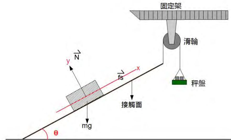
圖 42 實驗示意圖
