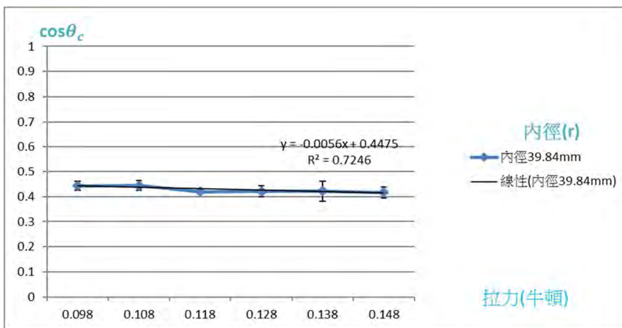
圖 47 \cos \theta_c 與拉力大小之關係圖
