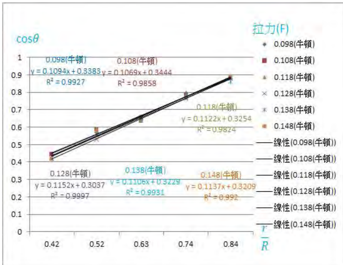
圖 59 \cos\theta_c 與線軸內外徑比值之關係圖(總和)
