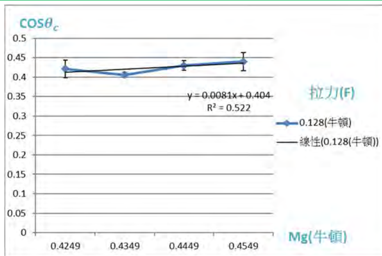
圖63 \cos \theta_c 與線軸重量之關係圖
