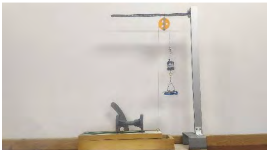
圖 40 將線軸直放於接觸面上
