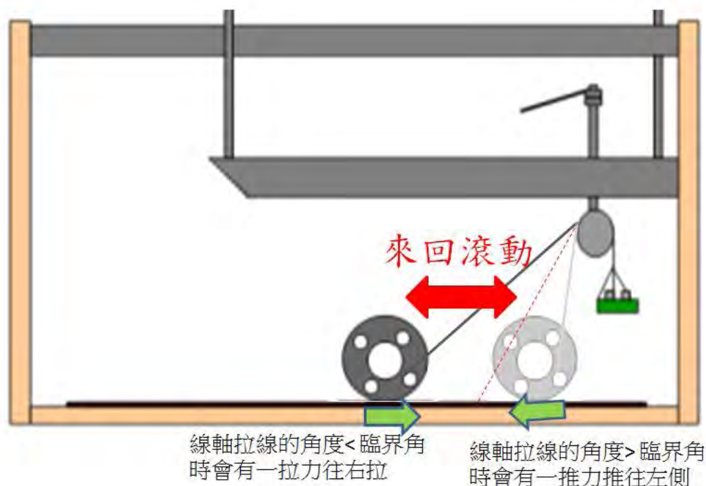
圖 77 實驗示意圖
