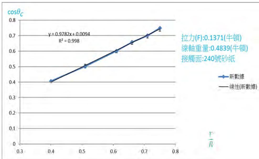
圖93實驗數據圖
