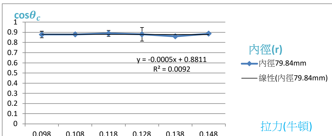
圖 51 \cos \theta_c 與拉力大小之關係圖
