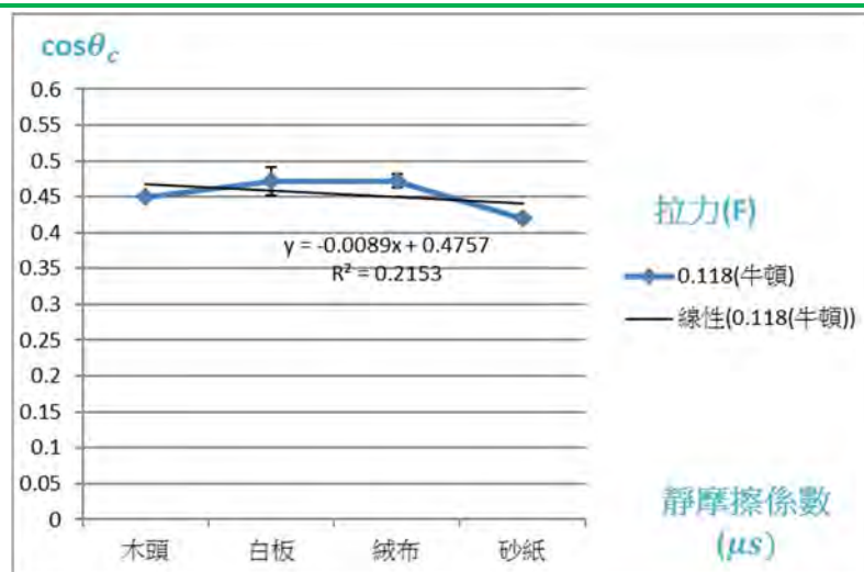
圖69 \cos \theta_c 與靜摩擦係數之關係圖
