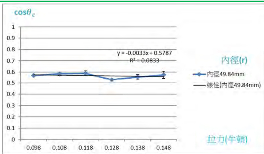
圖 48 \cos \theta_c 與拉力大小之關係圖
