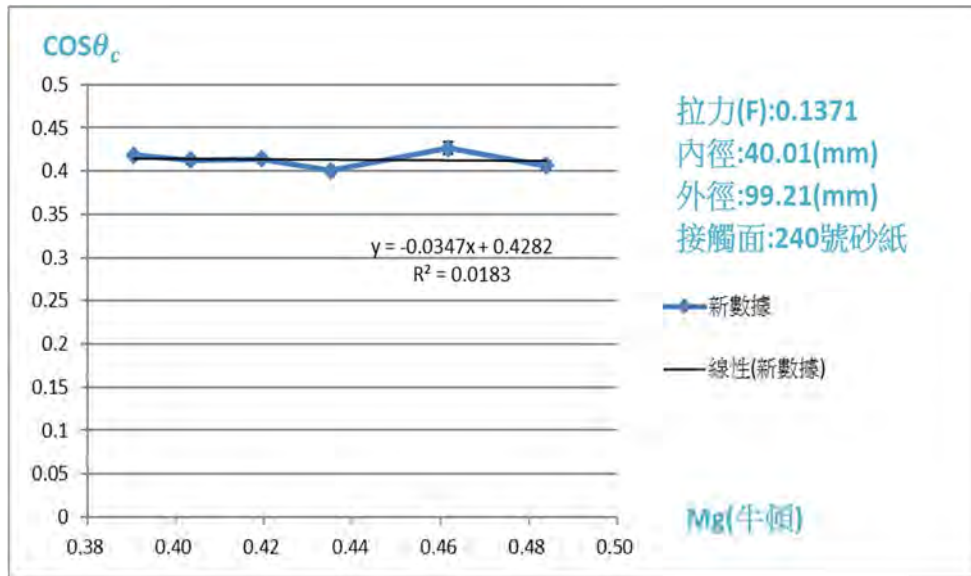
圖 92 實驗數據圖
