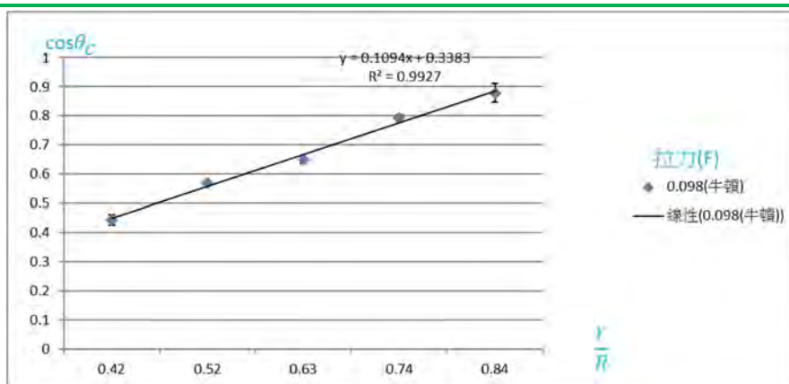
圖53 \cos \theta_c 與線軸內外徑比值之關係圖
