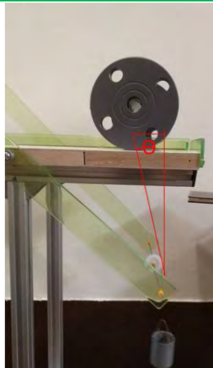
圖 75 下方臨界角
