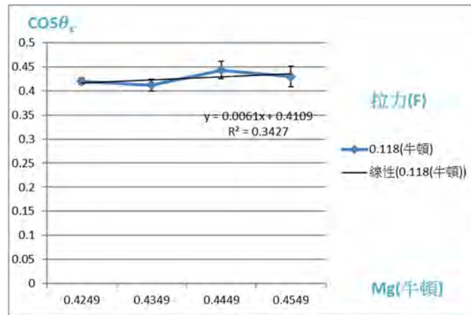
圖62 \cos \theta_c 與線軸重量之關係圖
