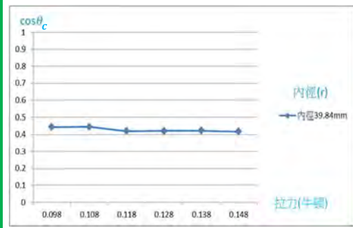
圖 32 將彙整之 \cos\theta_c 值做成關係圖
