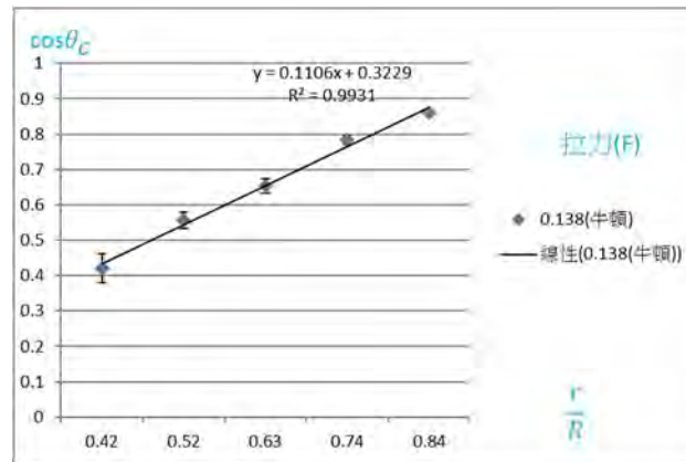
圖57 \cos \theta_c 與線軸內外徑比值之關係圖
