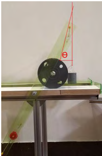
圖 74 上方臨界角
