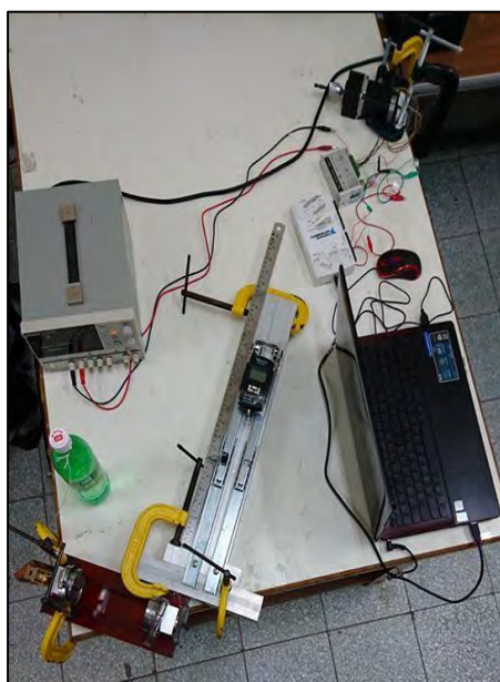
(圖二)儀器架設全貌圖
