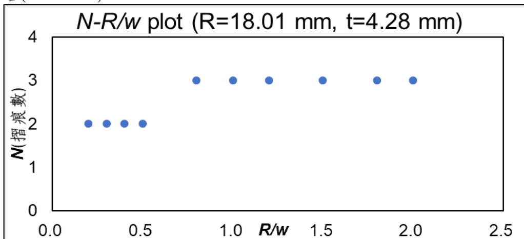
(圖三十四)厚度不容忽視( t=4.28 mm)之水管半徑、長度比值與摺痕數關係圖
