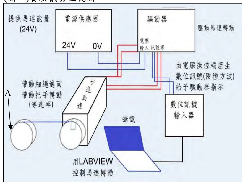
(圖三)儀器架設示意圖，圖一和圖三的 A 構造相同
