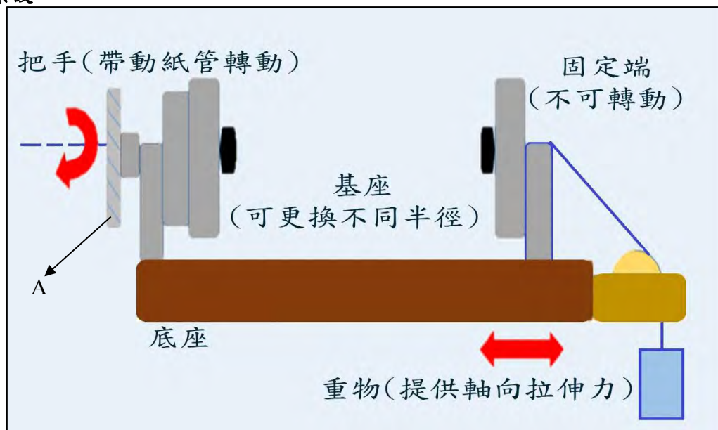
(圖一)實驗儀器正視圖
