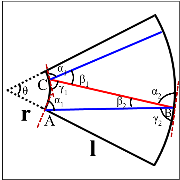
(圖二十三)大小管平面圖幾何模型(凹痕(藍)、凸痕(紅))
