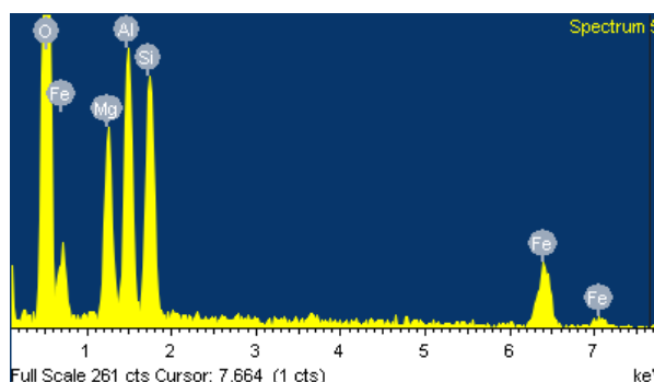
圖 4-22 EDS 分析黛綠色螺溪石中所含的金屬元素
