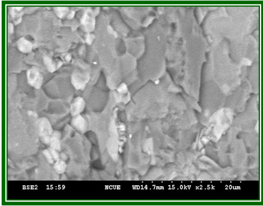
圖 4-3 SEM 底下放大 2500 倍的螺溪石礦物組成
