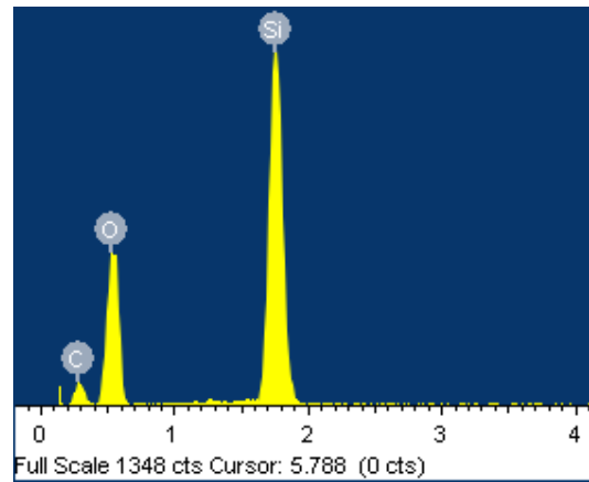
圖 4-5 螺溪石中片狀物質所含的金屬元素
