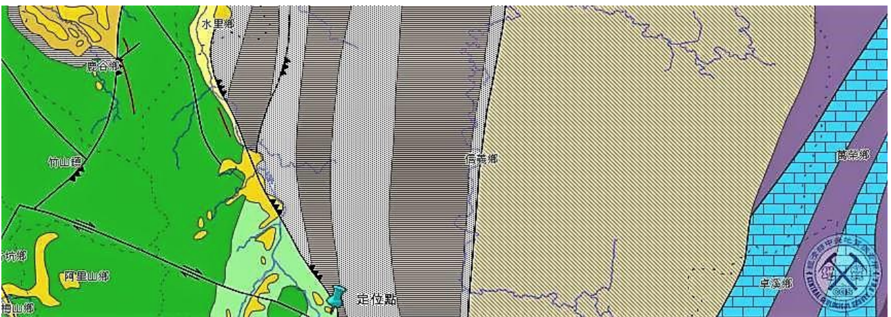
圖七 螺溪石礦脈的分布：東埔村人倫山
