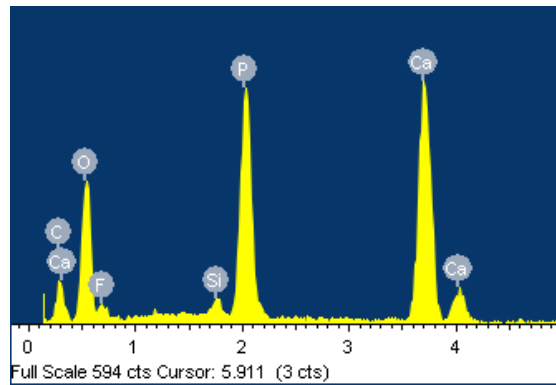
圖 4-7 螺溪石中顆粒狀物質所含的金屬元素
