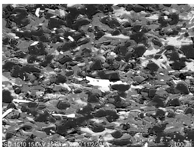
圖 4-8-1 SEM 底下放大 400 倍的螺溪石礦物組成
