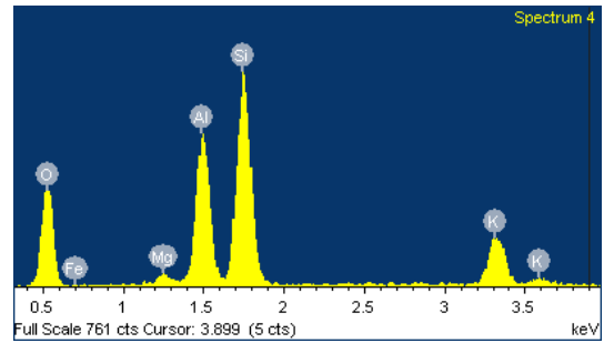
上圖 4-2 透過 EDS 分析螺溪石的組成物質
