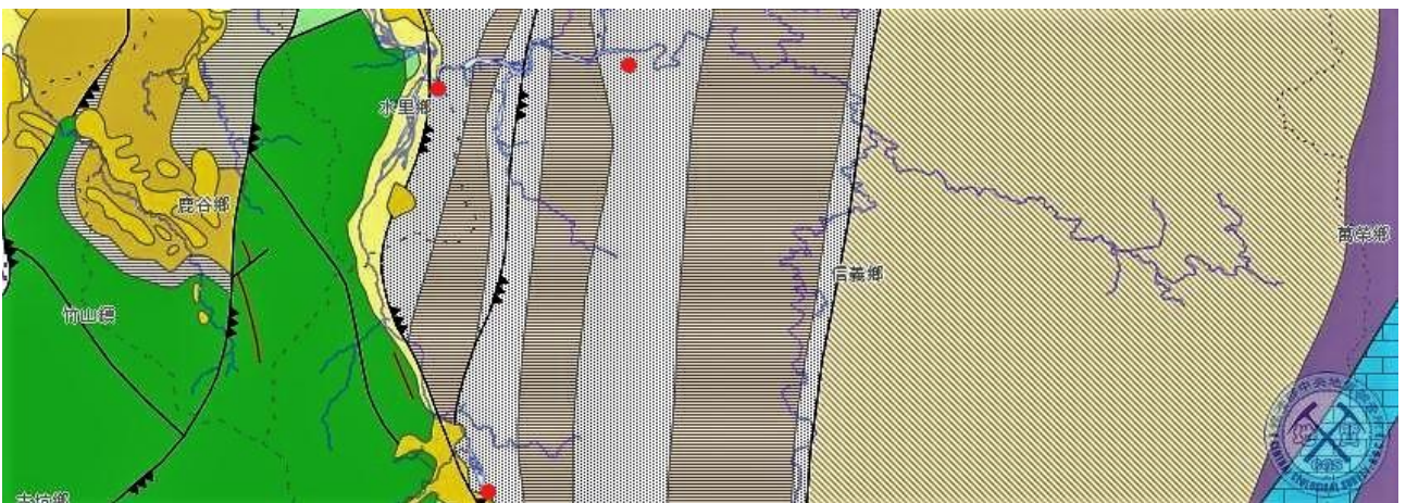
圖八 螺溪石礦脈分布的三角區域
