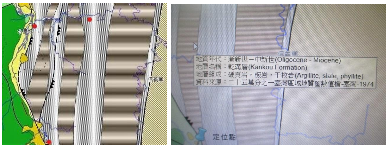
圖 3-6-1：螺溪石岩脈分布的三角地帶 圖 3-6-2：螺溪石岩脈的地質年代與地層名稱
