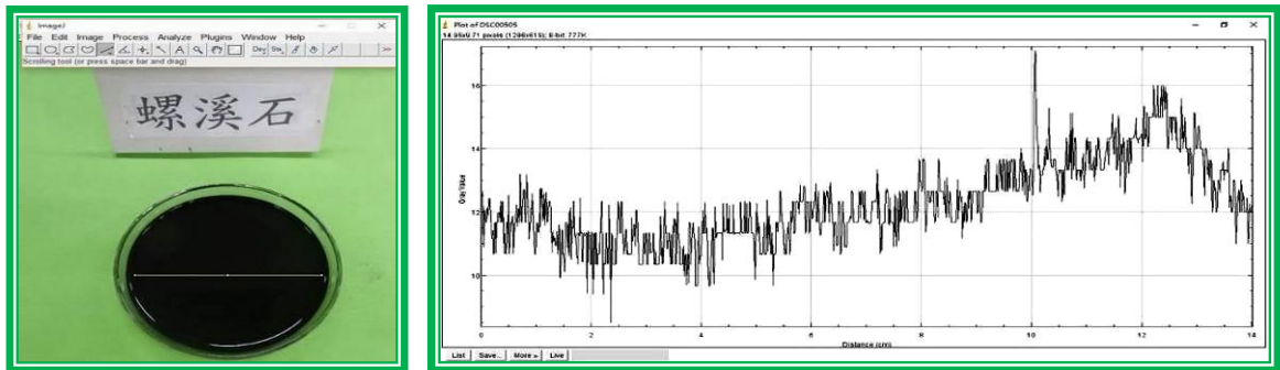
圖 3-22 墨液的成色分析 (1)我們先將墨液置於培養皿中，拍攝墨液照片，將照片於 imageJ 中計算其灰度值，最後將灰度值，轉換成「 墨黑度 」。(2)計算出各點墨黑度後，取其平均，代表該墨液的平均墨黑度。
