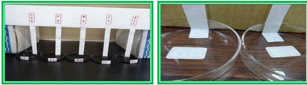
圖 3-21 墨液吸附實驗 本組將宣紙剪成長 20cm，寬 2cm 的長條狀，並固定在培養皿內的面積，以確保吸附墨液的面積固定。隨後記錄宣紙上墨液上升的高度，進行墨液吸附力的比較。
