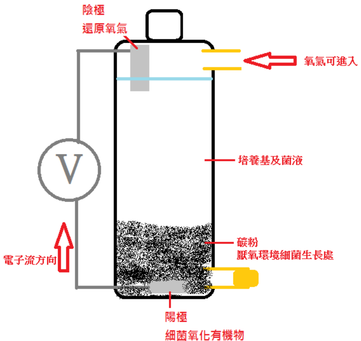
第一代裝置示意圖---單槽式結構
