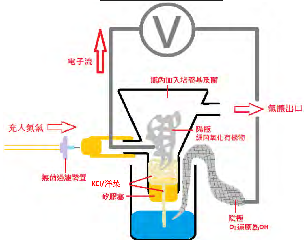
第二代裝置示意圖
