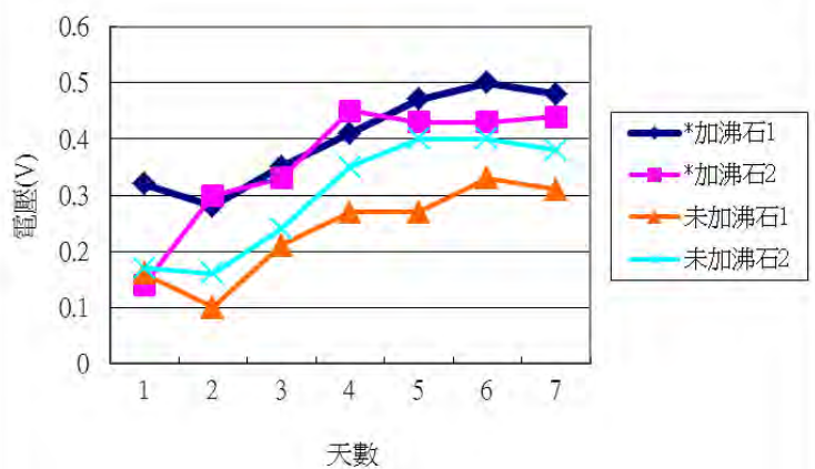
三代裝置4槽一週電壓變化
