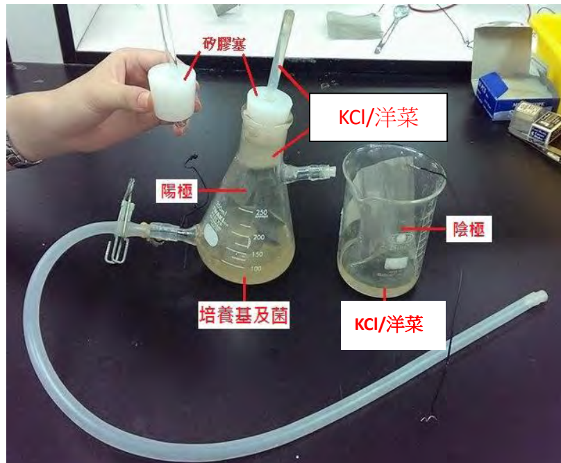
第二代裝置及其分解圖
