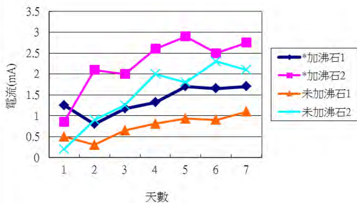
三代裝置4槽一週電流變化
