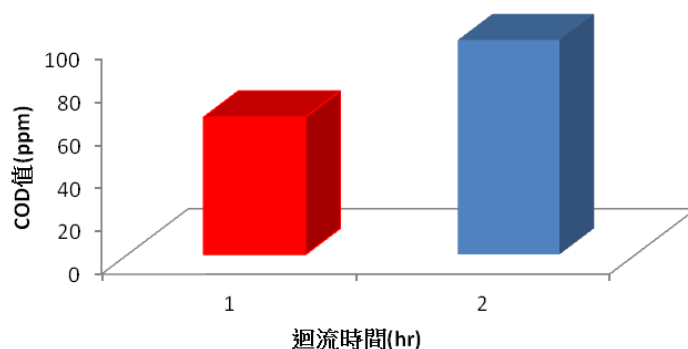
圖六(一)：傳統密閉式迴流法檢測 KHP COD 值
