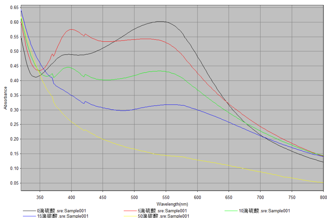
加入濃 \text{H}_2\text{SO}_{4(\text{aq})} 的 UV-Vis 吸收光譜
