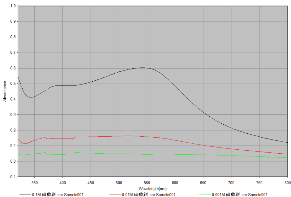
2 天後 UV-Vis 吸收光譜
