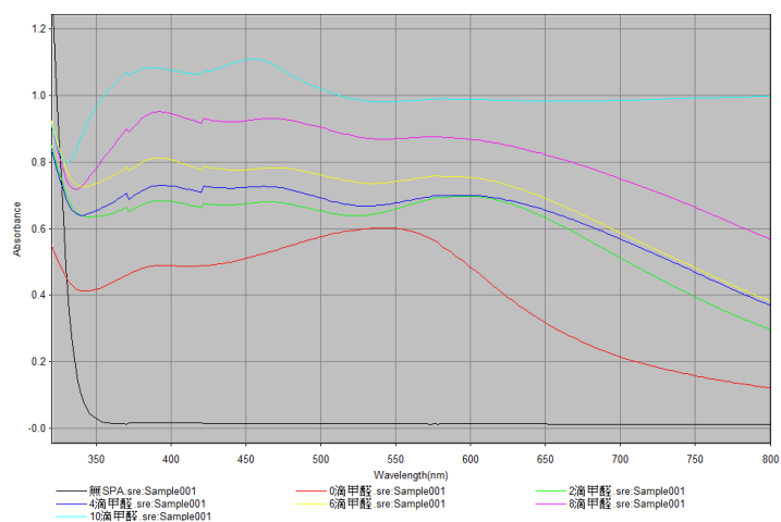
2 天後 UV-Vis 吸收光譜
