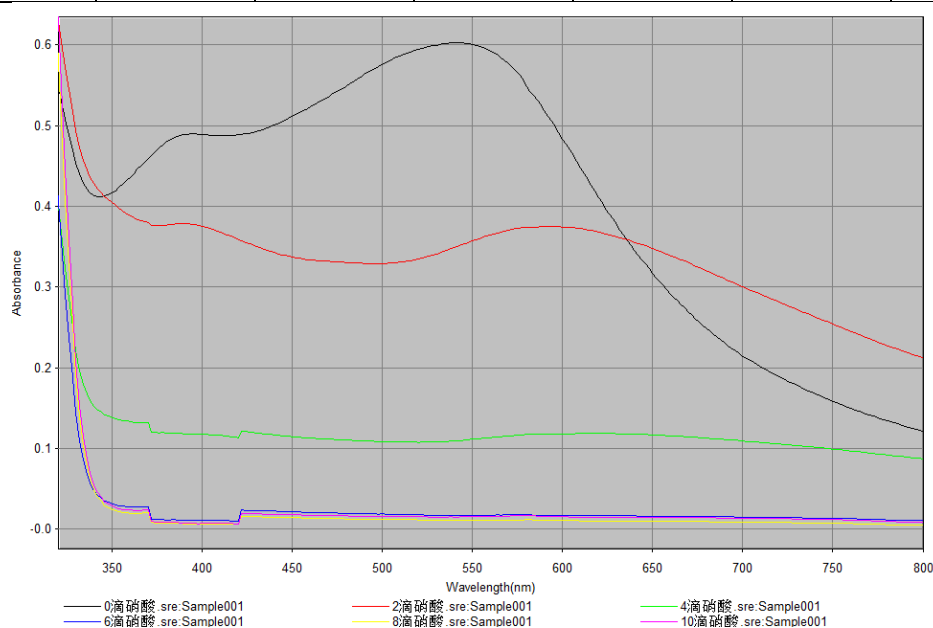
2 天後 UV-Vis 吸收光譜
