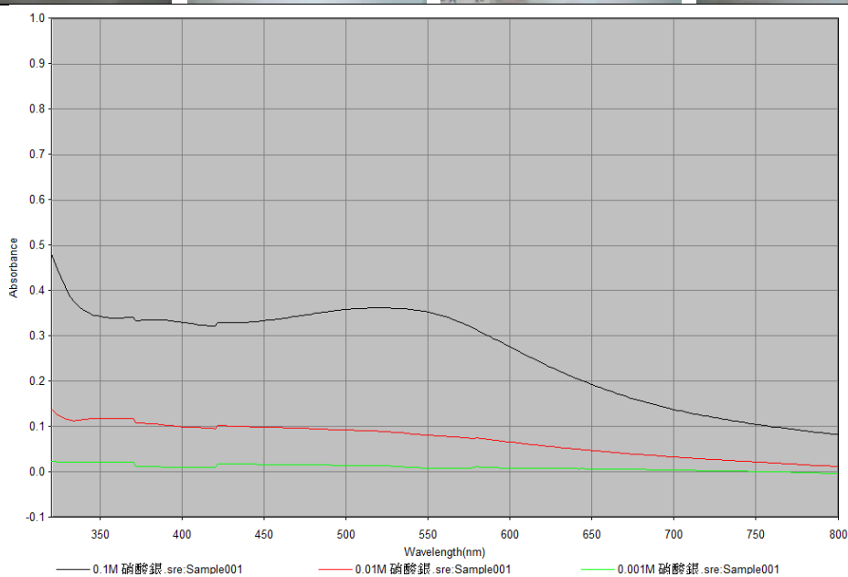
1 天後 UV-Vis 吸收光譜
