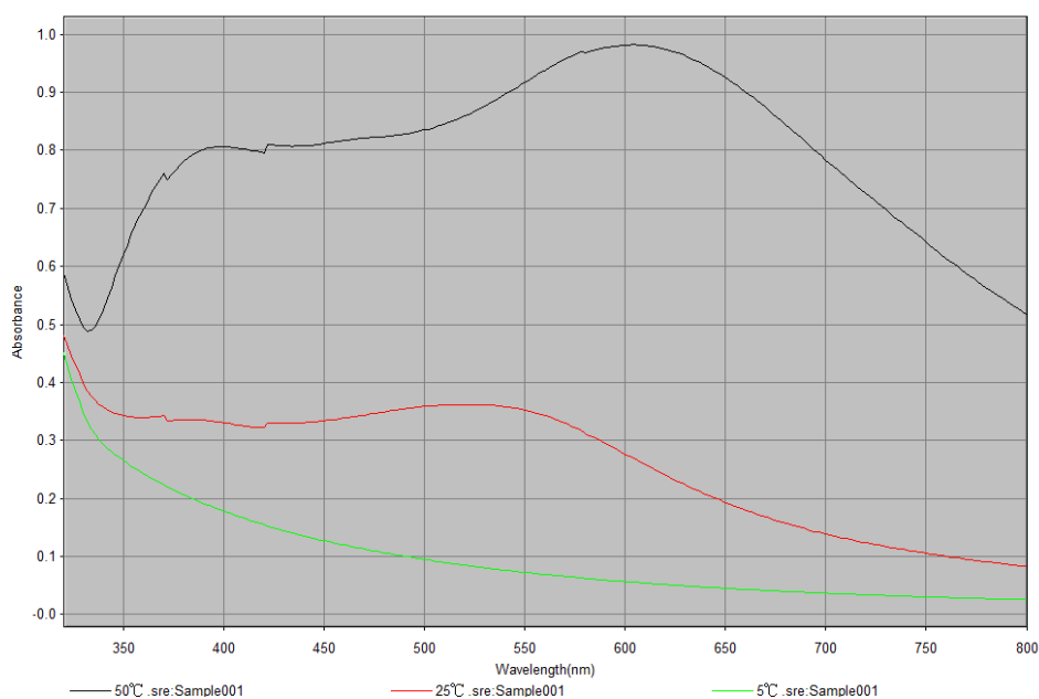
1 天後 UV-Vis 吸收光譜
