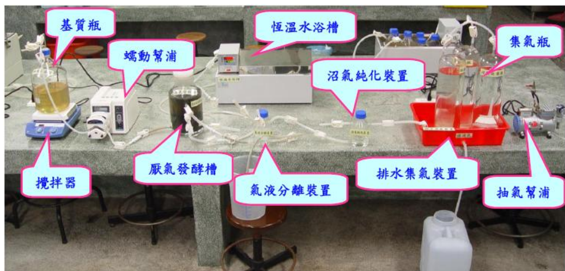
圖 2. 沼氣厭氣發酵裝置
