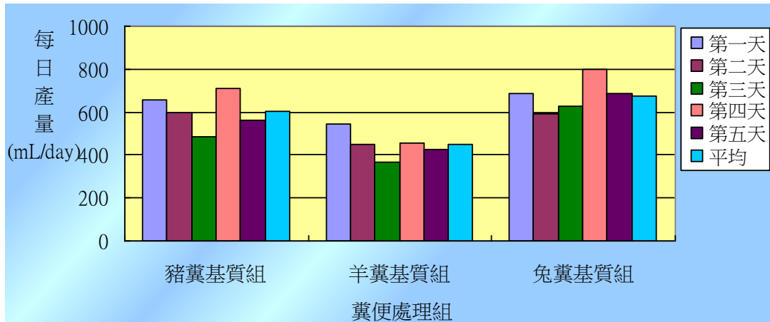
圖 27. 各種基質處理組沼氣每日產量比較圖
