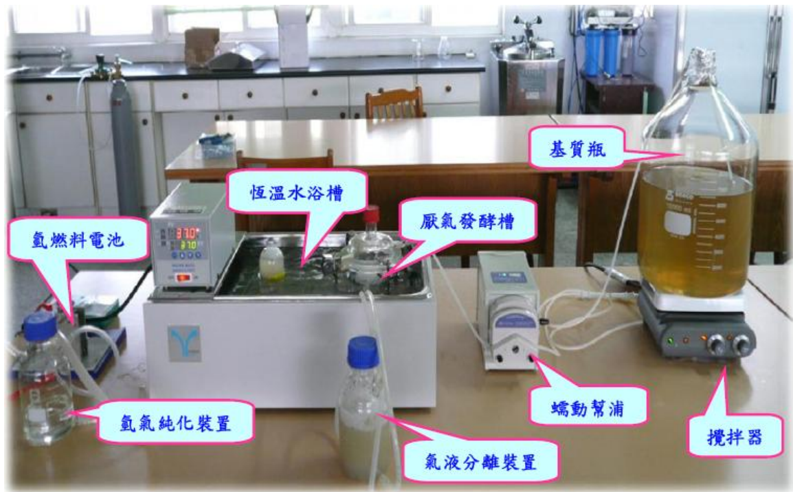
圖 1. 厭氣發酵產氫裝置圖
