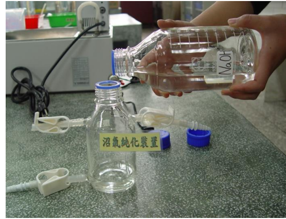
圖 19. 將 NaOH 倒入氣體純化裝置
