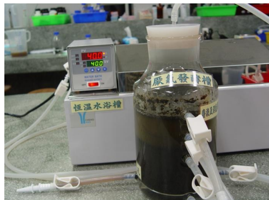
圖 17. 將產沼氣厭氧發酵槽定溫 40°C
