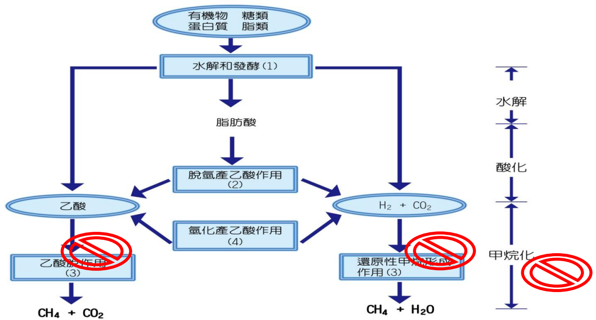
圖 8. 微生物產氫發酵的一般路徑
