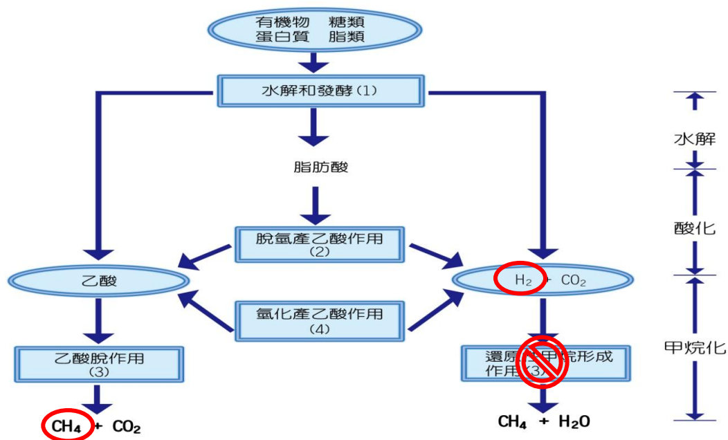
圖 24. 微生物產氫與沼氣發酵的結合
