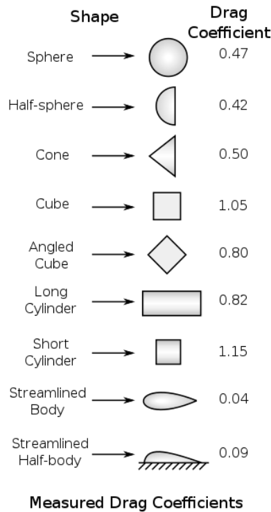
圖 6-1。不同形狀之阻力係數
