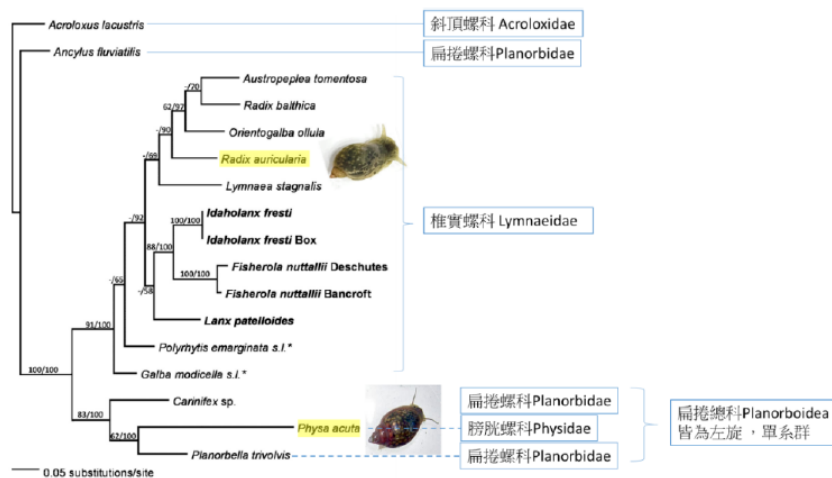
圖 1-6。根據 David C. Campbell, 2017 的研究結果更改繪製，前人以 16srRNA 序列建構淡水螺的親緣關係。囊螺學名 Physella acuta ，台灣椎實螺學名 Radix swinhoei ( Radix auricularia )。
