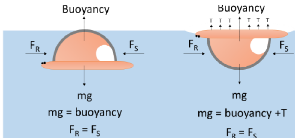
圖 3-8。漂浮與仰泳過程受力圖。阻力(FR)、進行動力(FS)、表面張力(T)、重量(mg)、浮力(buoyamcy)。
