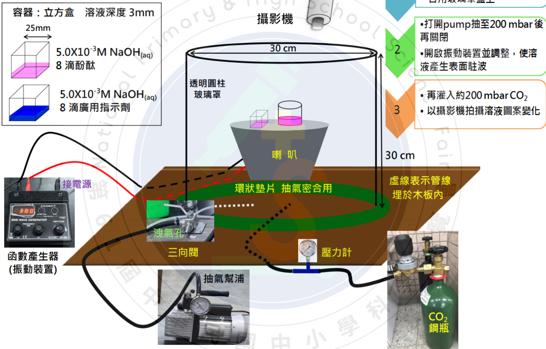
圖4-7 酸鹼溶液振動實驗裝置圖
