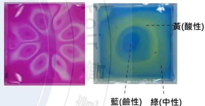
圖1-3 酸鹼反應+物理駐波
