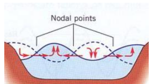
圖 4-4 液體之一維駐波示意圖[4]
