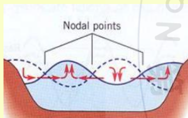
圖4-3 一維駐波示意圖
