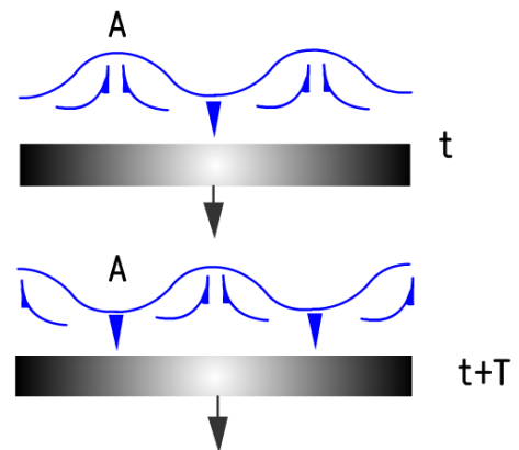
圖 4-6 法拉第駐波示意圖[2]
