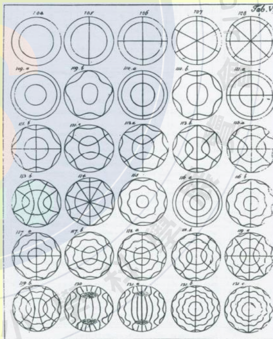
圖4-5 方板及圓板振動之克拉德尼圖案[4,5]
