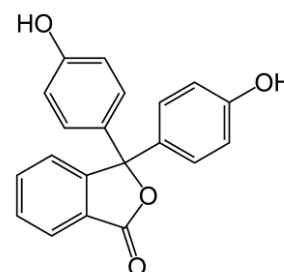
圖 4-2 酚酞結構圖
