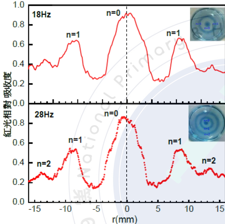
圖6-5 實驗五之藍瓶反應溶液經18Hz、28Hz共振3分後，紅光相對吸收度沿徑向之分布圖
