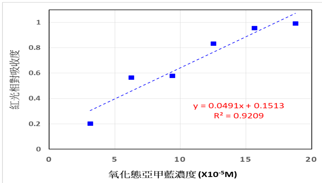
圖 6-12 氧化態亞甲藍濃度-紅光強度之檢量線
