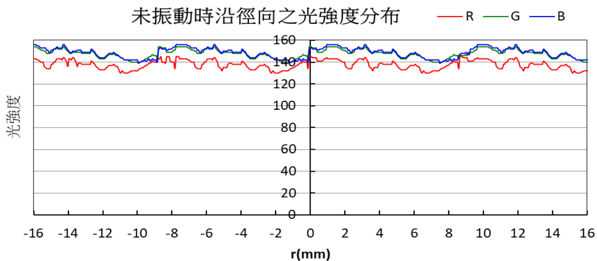
圖 6-6 實驗五之藍瓶反應溶液未振動時沿徑向之 RGB 數值分布圖
