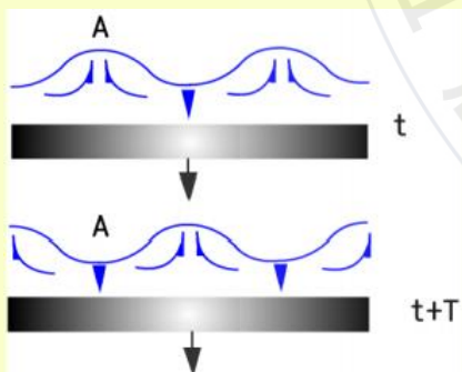
圖4-4 法拉第波示意圖[3]
