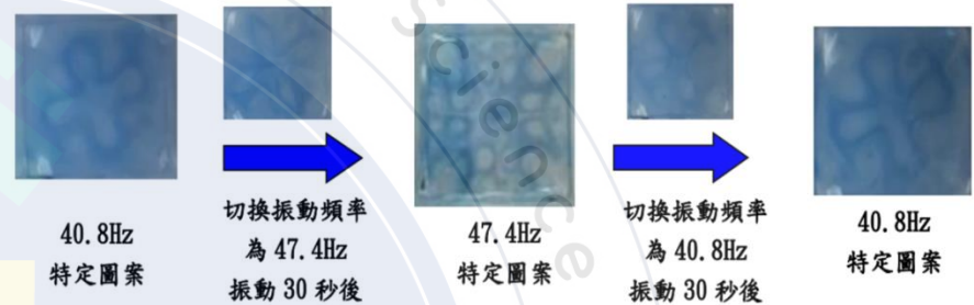
圖6-3 藍瓶反應溶液之振動圖案在2種特定頻率轉換後，仍可對應該頻率特定圖案之情形
