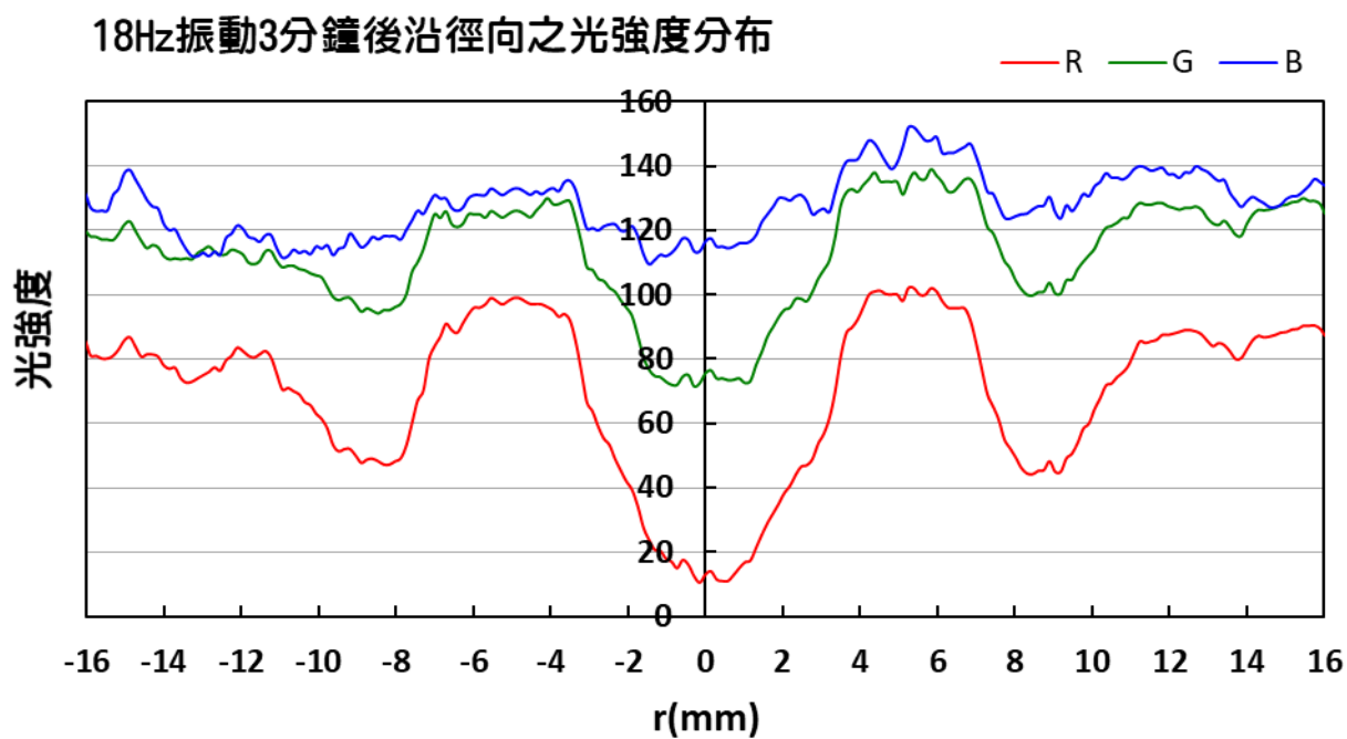
圖 6-7 實驗五之藍瓶反應溶液以 18Hz 振動 3 分鐘後沿徑向之 RGB 數值分布圖
