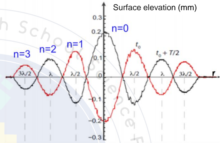
圖6-6 同心圓駐波沿徑向(r)之液體表面起伏情形
