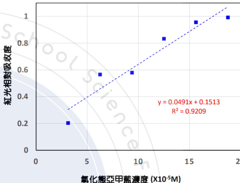
圖6-8 氧化態亞甲藍濃度-紅光相對吸收度之檢量線
