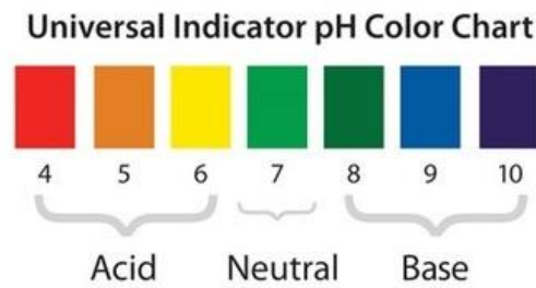
圖 4-3 廣用試劑變色範圍
