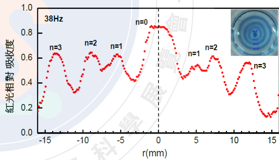
圖6-7 實驗五之藍瓶反應溶液經38Hz共振3分鐘後，紅光相對吸收度沿徑向之分布圖
