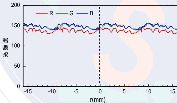
圖6-4 左：實驗五之藍瓶反應溶液未振動 右：18Hz共振3分後沿徑向之RGB數值分布圖
