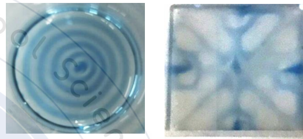
圖1-2 藍瓶反應溶液+物理駐波
