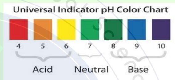
圖4-2 廣用試劑酸鹼顏色變化對照圖
