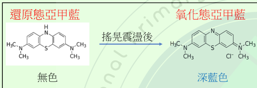
圖4-1 藍瓶溶液反應說明圖
