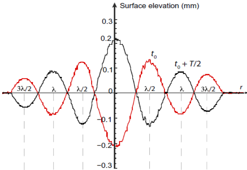
圖 6-9 同心圓駐波沿徑向( r )之液體表面起伏情形
