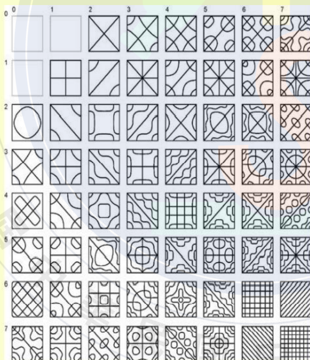
圖4-5 方板及圓板振動之克拉德尼圖案[4,5]
