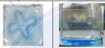
圖 6-2 振動時的亞甲藍之溶液 (左)俯視圖 (右)側視圖
