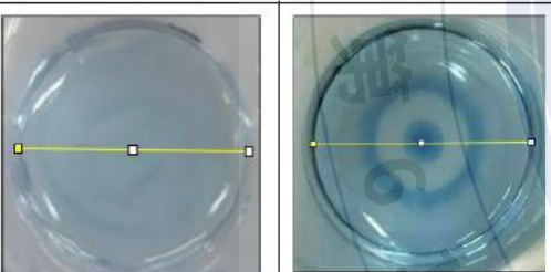
圖6-5 a.未振動前沿徑向分析 b. 18Hz共振後，沿同一徑向分析
