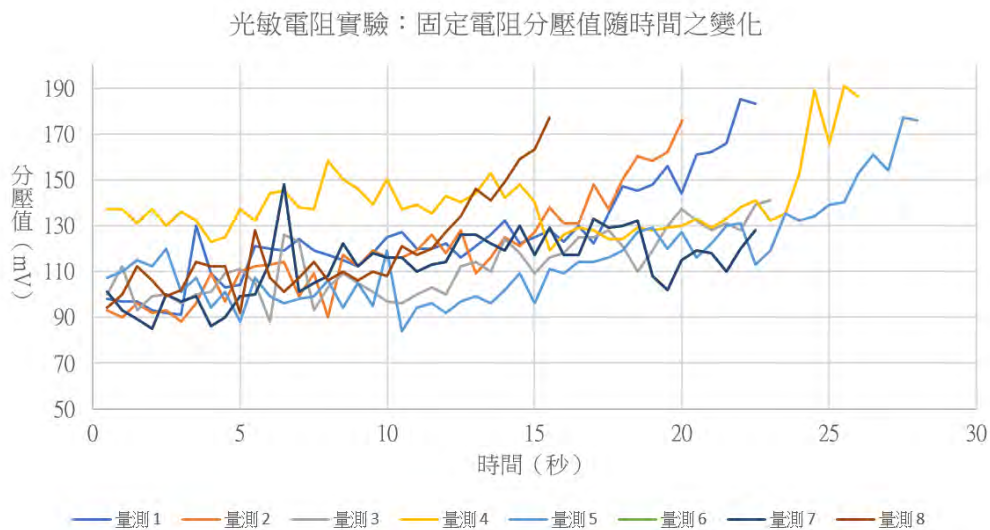
圖 16 有遮光罩情況下，光敏電阻偵測器實驗中固定電阻分壓隨時間之變化，趨勢類似圖 15 中結果
