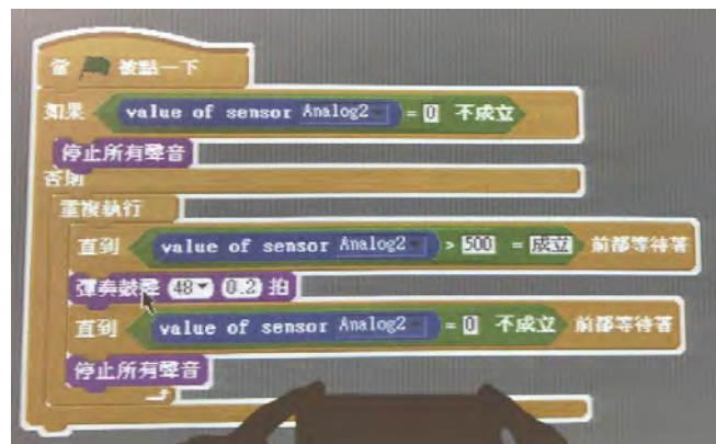
圖 13 利用水銀開關的導通與否偵測水位臨界值之程式
