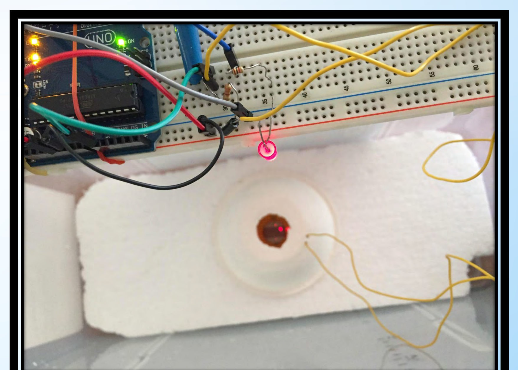
光敏電阻加遮光罩實驗
