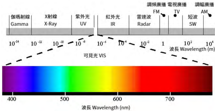
圖 23 光譜分布區間圖（參考資料 4）
