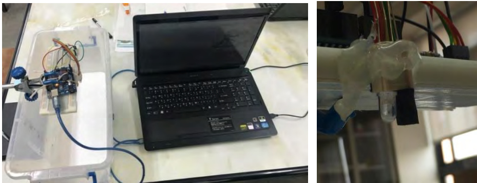
圖 8 (左) 利用紅外線訊號接收強度偵測水位高度系統實體圖 (右) 於紅外線接收器外加上黑色光罩可減少環境紅外線影響
