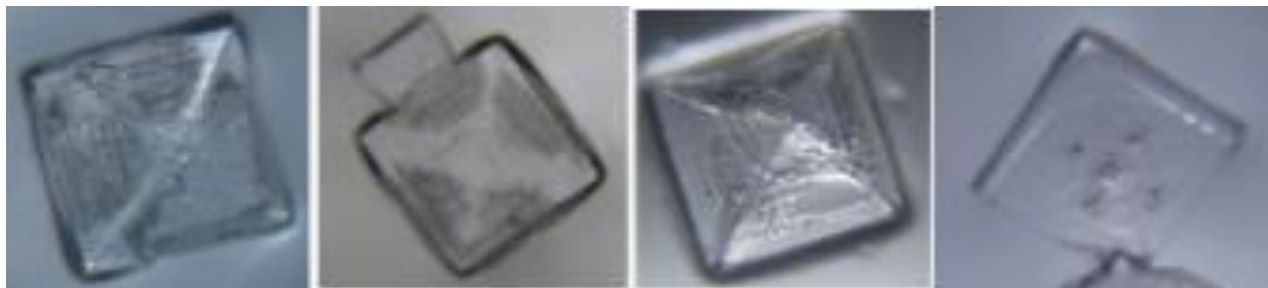
圖 29：不同情況下產生的食鹽晶體表面的階梯螺旋紋。左一，左二：溶質供應充足，產生中央隆起的階梯螺旋紋丘。右一，右二：溶質供應不足，產生中央凹陷的階梯螺旋紋谷。
