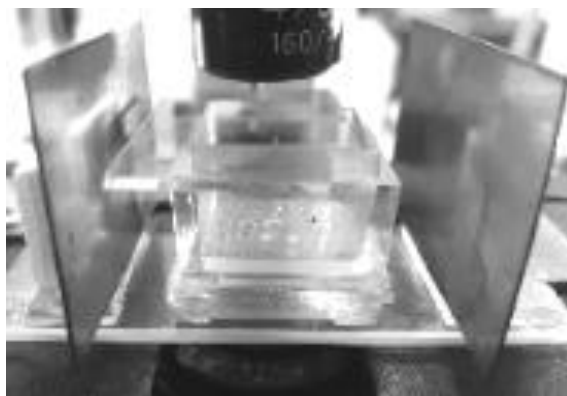
圖 36：研究 3-1 顯微鏡下，高電壓平行電場的液滴晶體成長實驗裝置（第三階段）
