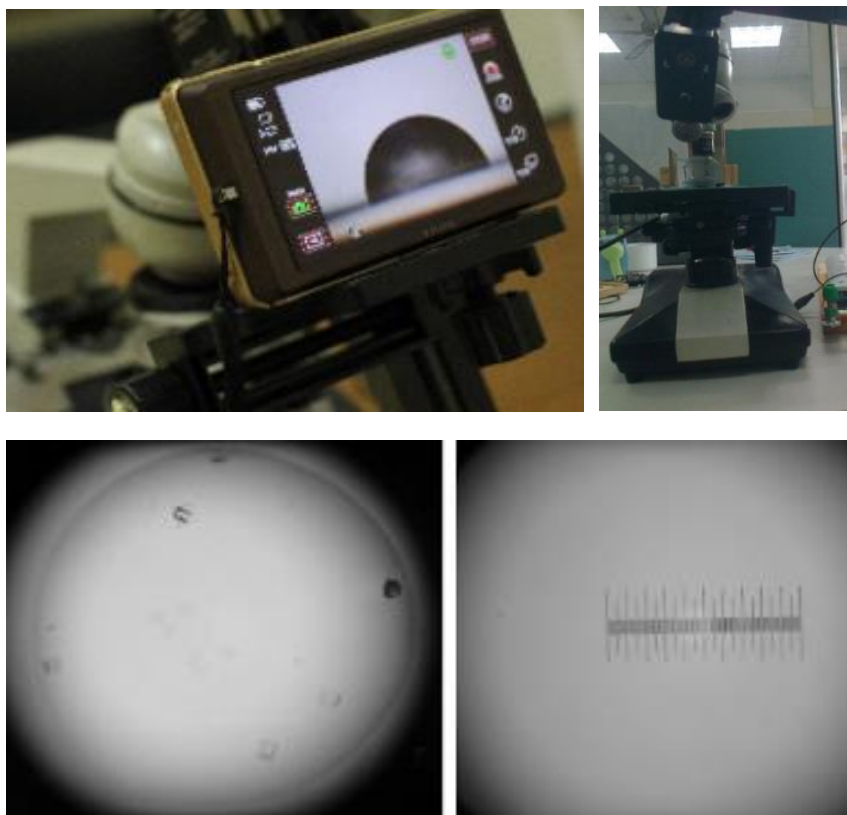
圖 09：第四代裝置：相機-複式顯微鏡的連接（左上）與鏡座上的玻璃座平行銅片電場（右上），水珠視野範圍（左下），與相同顯微鏡倍數下的載玻片測微尺（右下），用來估算晶體尺寸。
