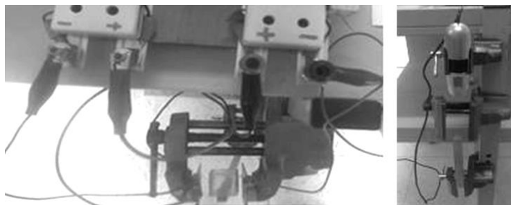
圖 04：高電壓裝置連接木工固定架平行銅片電場（左）與可攜式電子顯微鏡的擺法（右）。
