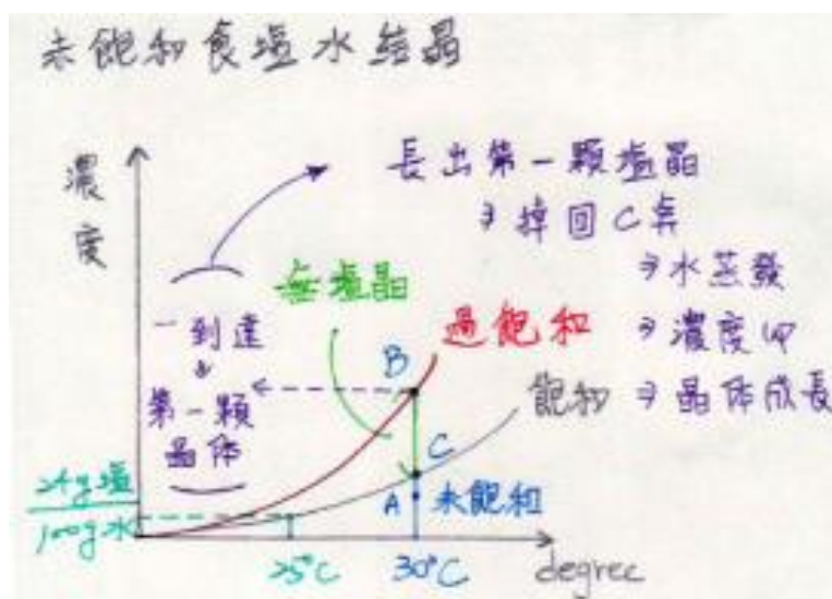
圖 27：食鹽水結晶溶解度曲線、過飽和度曲線與濃度變化示意圖
