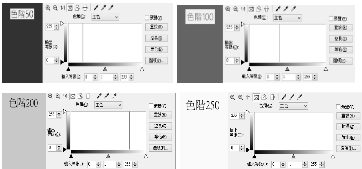
圖 07：photoimpact 色階設定分佈圖
