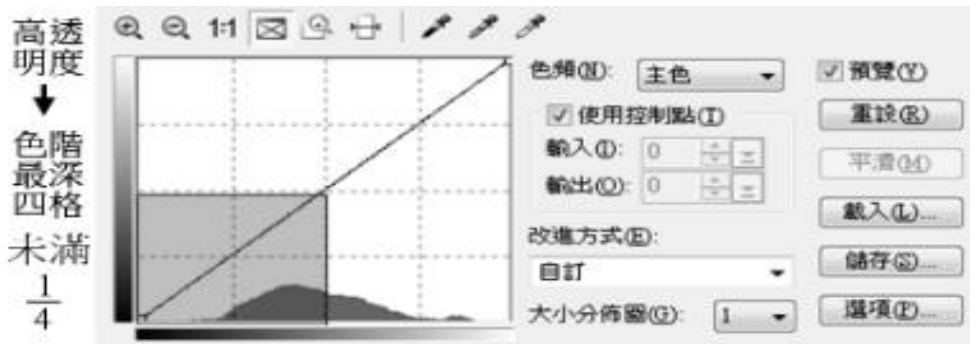
圖 08：photoimpact 色階分佈判斷透明度
