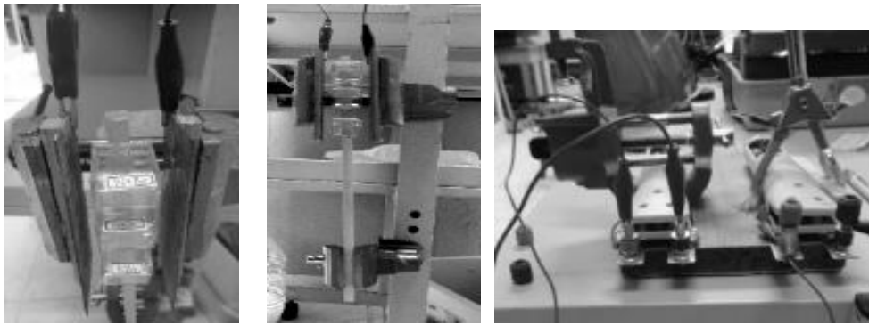
圖 05：撤去可攜式顯微鏡的第三代裝置, 在平行電場中一次可做三種不同變因實驗
