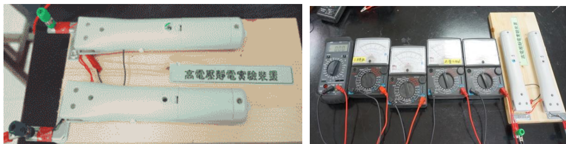
圖 02：高電壓裝置 (左) 與裝置接上串聯後的三用電表，測量其電壓 (右)。
