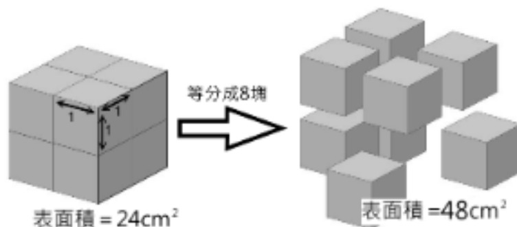
圖 28：國中課本中有關表面積與顆粒大小關係的示意圖
