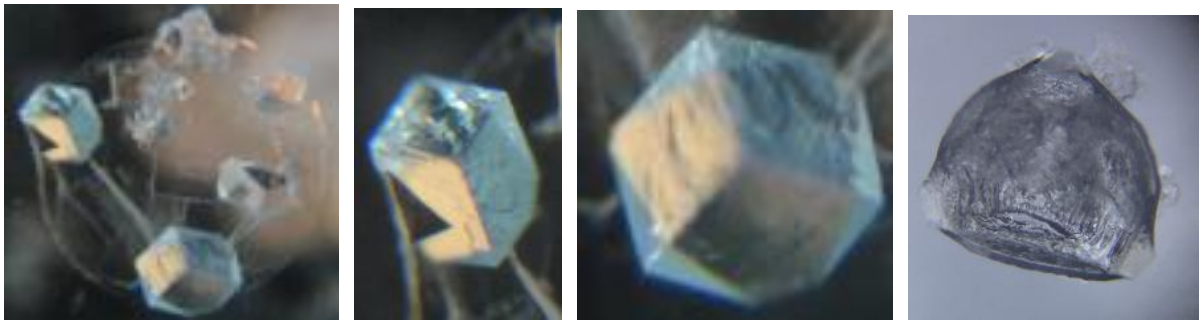
圖 45:有施加高電壓平行電場的食鹽晶體,晶面不平行底座,容易誤判為晶形發生改變 左一:高電壓(4850 伏特)電場下,水珠中長出多顆晶體,可看出水珠原有邊界 左二:高電壓(4850 伏特)下,水珠中長出的傾斜長方體晶體 左三:高電壓(4850 伏特)下,水珠中長出的傾斜正立方體晶體 右一:在高倍率,低立體感的影像中,容易被誤判為晶形改變的傾斜立方晶體
