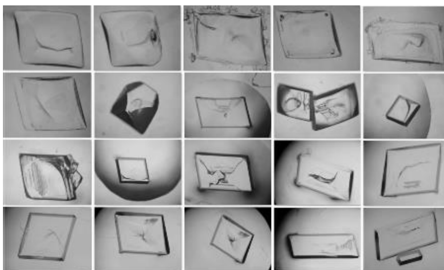
圖 54：顯微鏡下，無施加高電壓平行電場（電壓=0 伏特）的硝酸鈉液滴晶體成長影像
