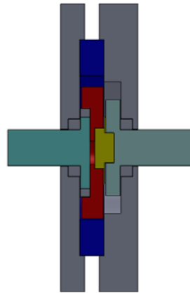
圖 15 電腦模擬立體圖和剖面圖
