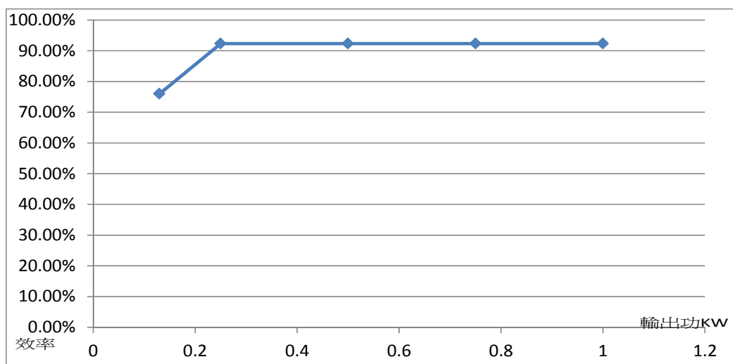
圖 26 齒輪式減速機效率曲線(輸入功率為變數)
