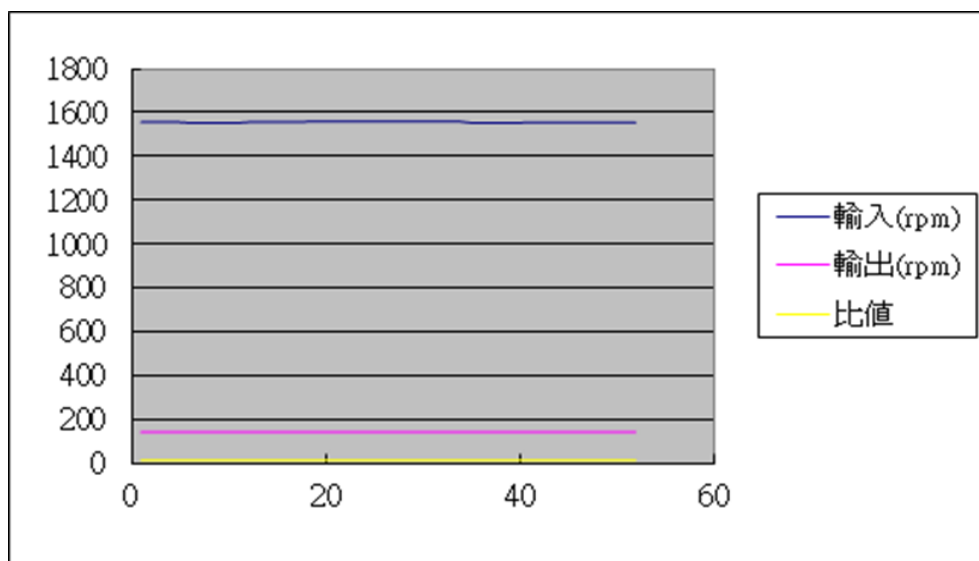
圖 25 隨機取樣圖表
