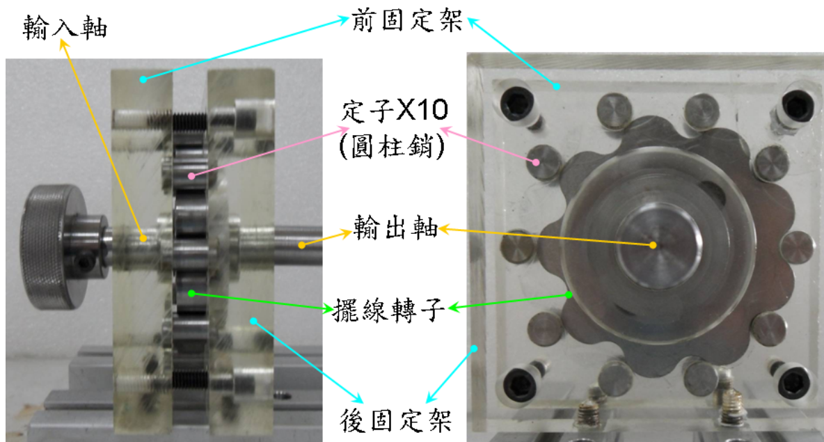
圖 23 擺線轉子減速機實體組合圖
