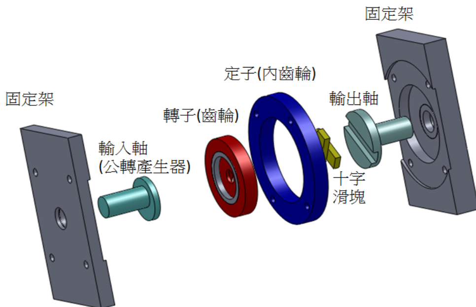
圖 14 內擺運動減速機之齒輪式零件爆炸圖
