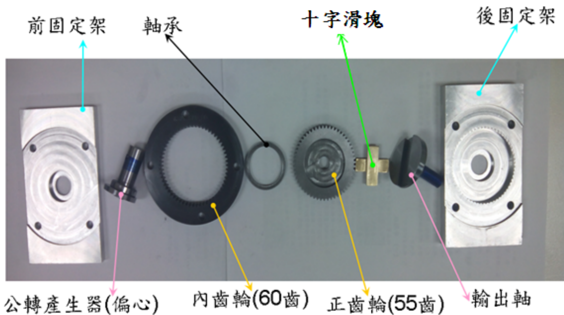
圖 16 實體零件圖
