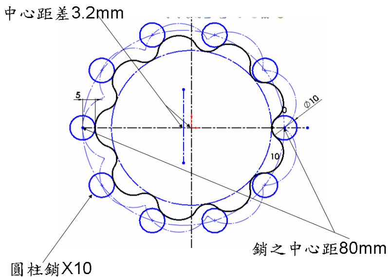
圖 4 10 顆銷的位置排列圖
