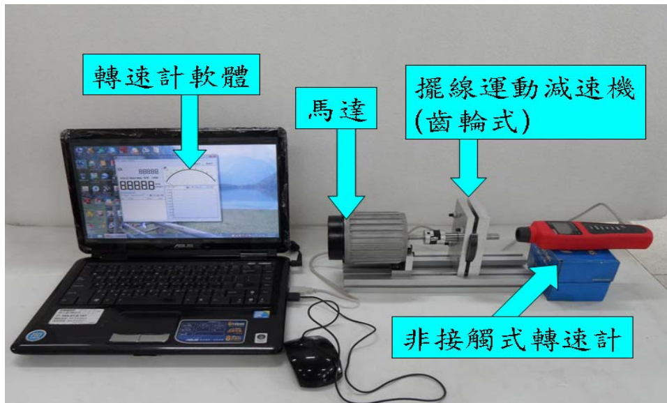
圖 24 測試平台(齒輪式)
