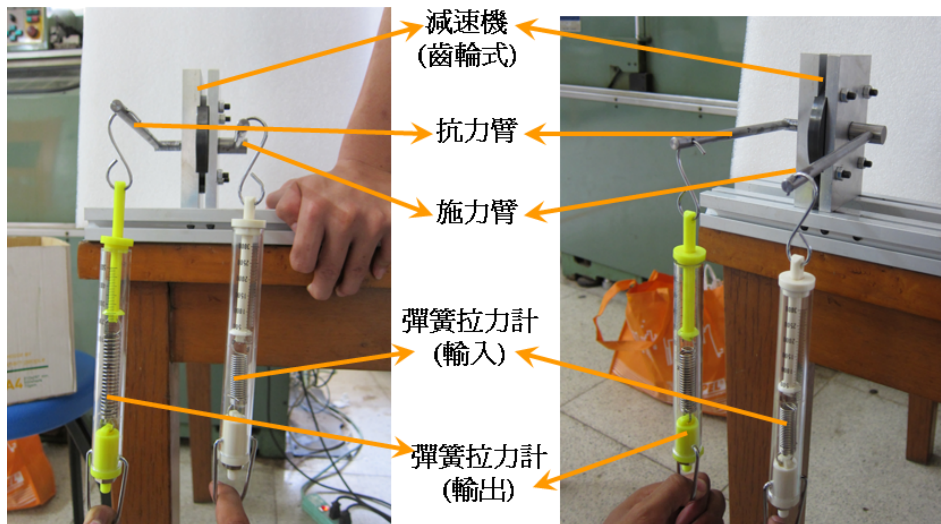
圖 27 效率測試情形
