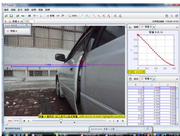
圖 14 使用 Tracker 測量開門時間
