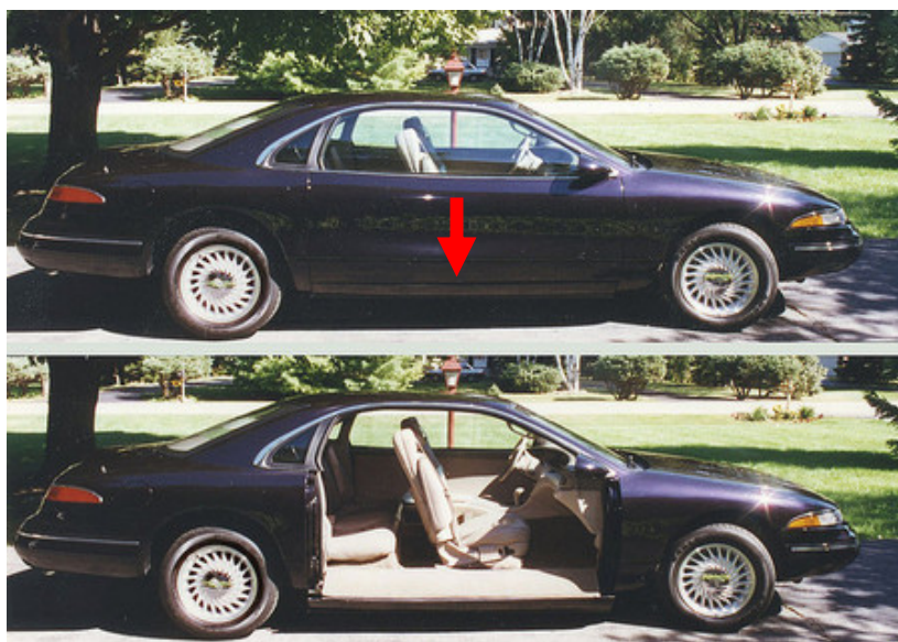
圖 6 車門向下開啟
