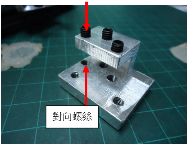
圖 58 新的門把固定設計使用對向螺絲
