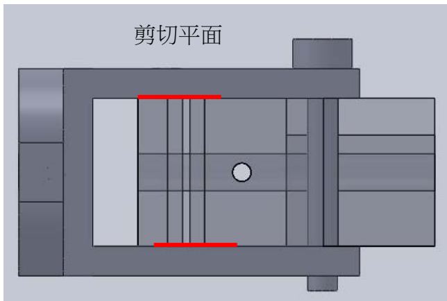
圖 37 安全鎖雙剪位置圖
