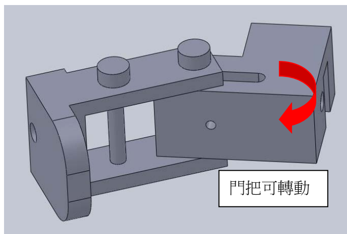
圖 23 零件組立圖
