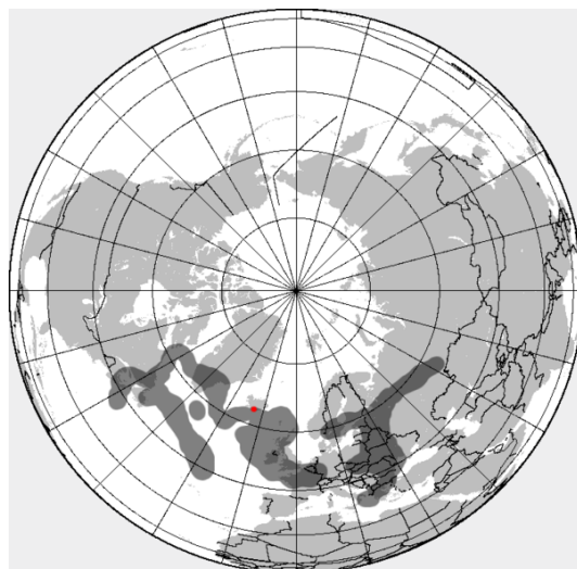
圖 12 2010 年 4 月 21 日火山灰雲分布
