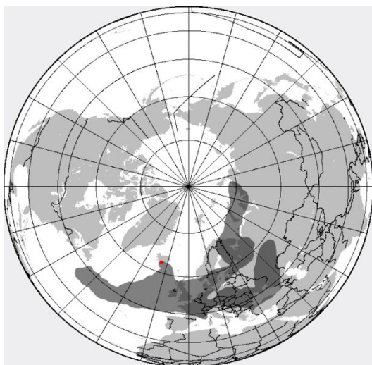
圖 9 2010 年 4 月 18 日火山灰雲分布
