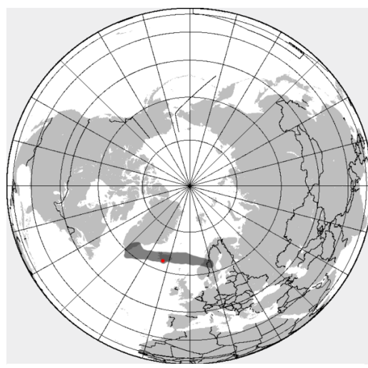
圖 16 2010 年 4 月 25 日火山灰雲分布
