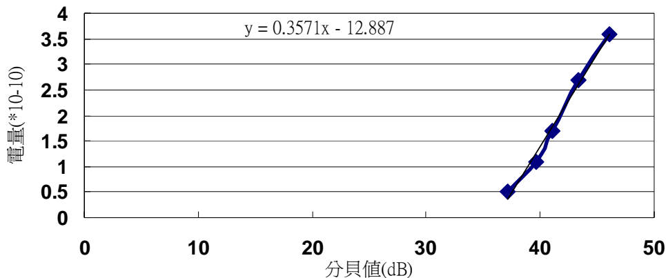
電量與分貝關係圖
