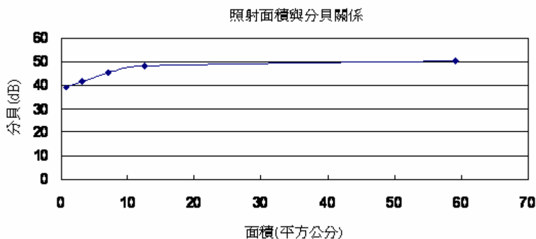
圖 21 照射面積與分貝值關係
