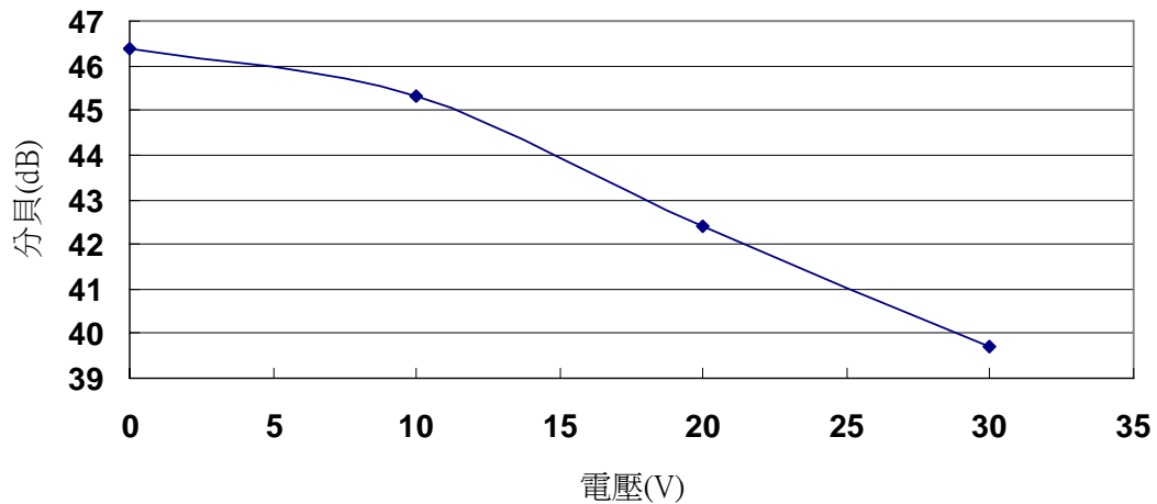
圖 13 碳黑於不同電壓中分貝值下降圖
