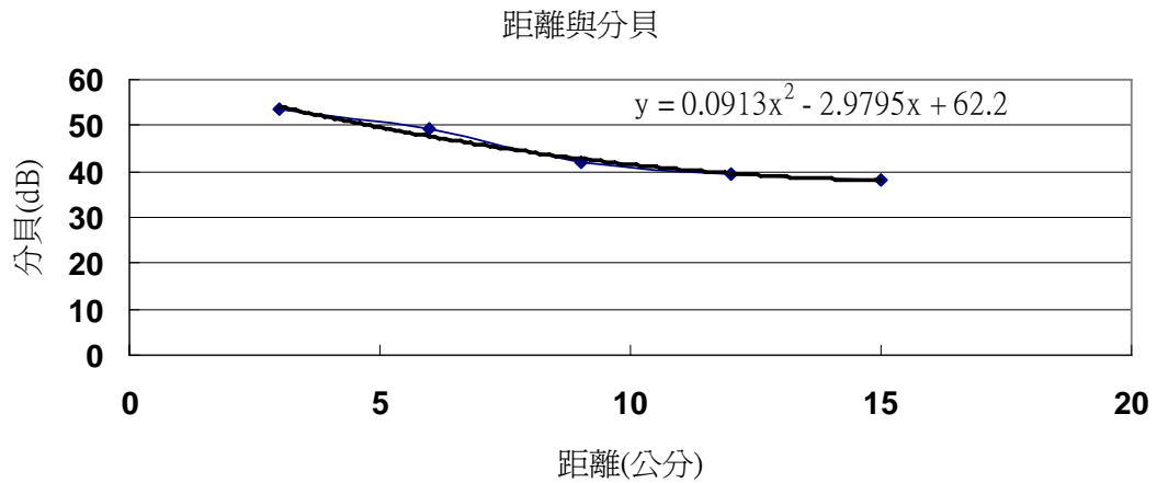
圖 17 距離與分貝值關係圖
