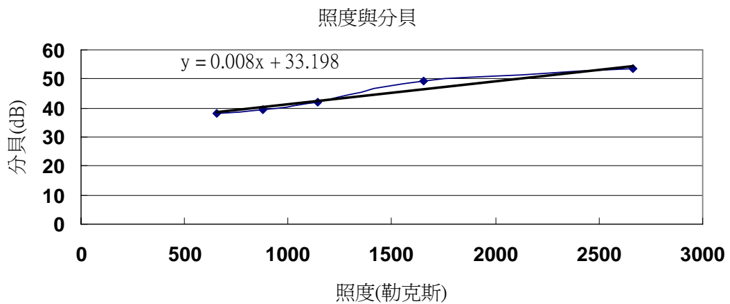
圖 18 照度與分貝值關係圖
