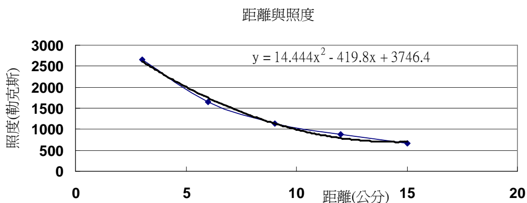
圖 16 距離與照度關係圖
