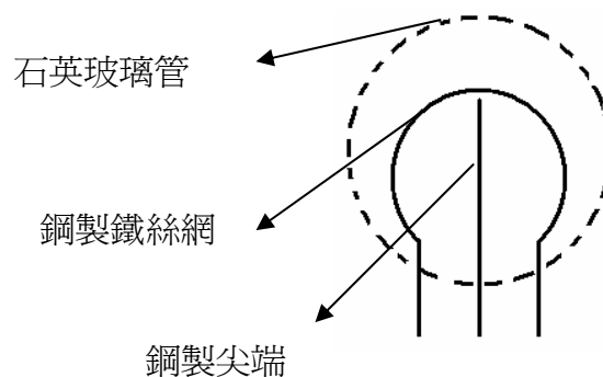
圖 7 光電管示意圖
