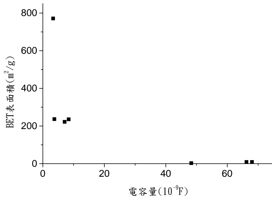
圖七 BET 表面積與電容量關係圖
