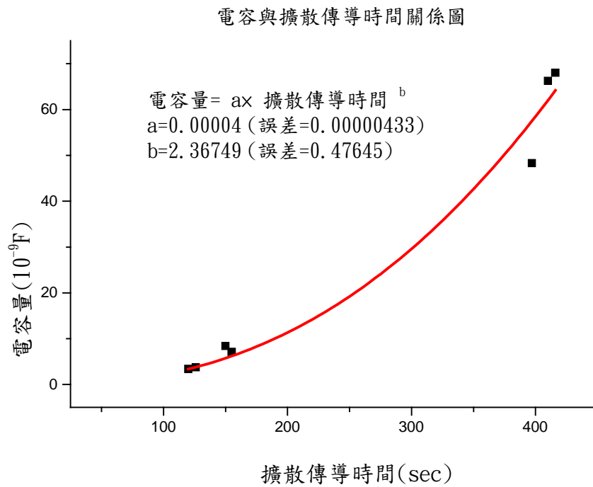
圖六、電容與擴散傳導時間關係圖
