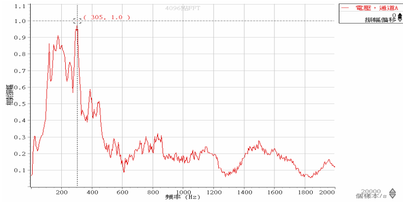
圖 22 同一顆未成熟西瓜二號拍擊點拍聲頻譜
