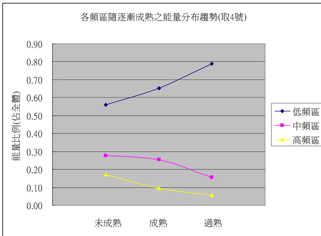
圖 14 隨成熟度之增加，各頻區之能量分佈變化圖（4 號拍擊點）
