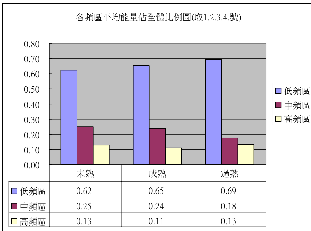
圖 15 不同類西瓜其各頻區之能量分佈圖（1-4 號拍擊點）
