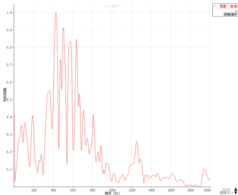
圖 8 加入水的皮球的主頻率
