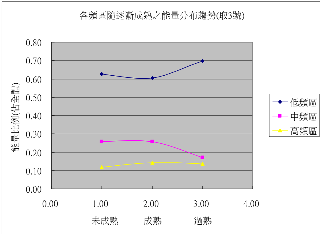
圖 13 隨成熟度之增加，各頻區之能量分佈變化圖（3 號拍擊點）
