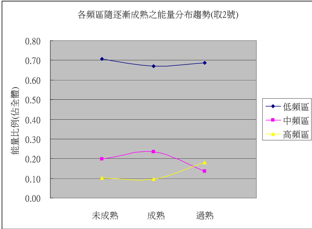
圖 12 隨成熟度之增加，各頻區之能量分佈變化圖（2 號拍擊點）
