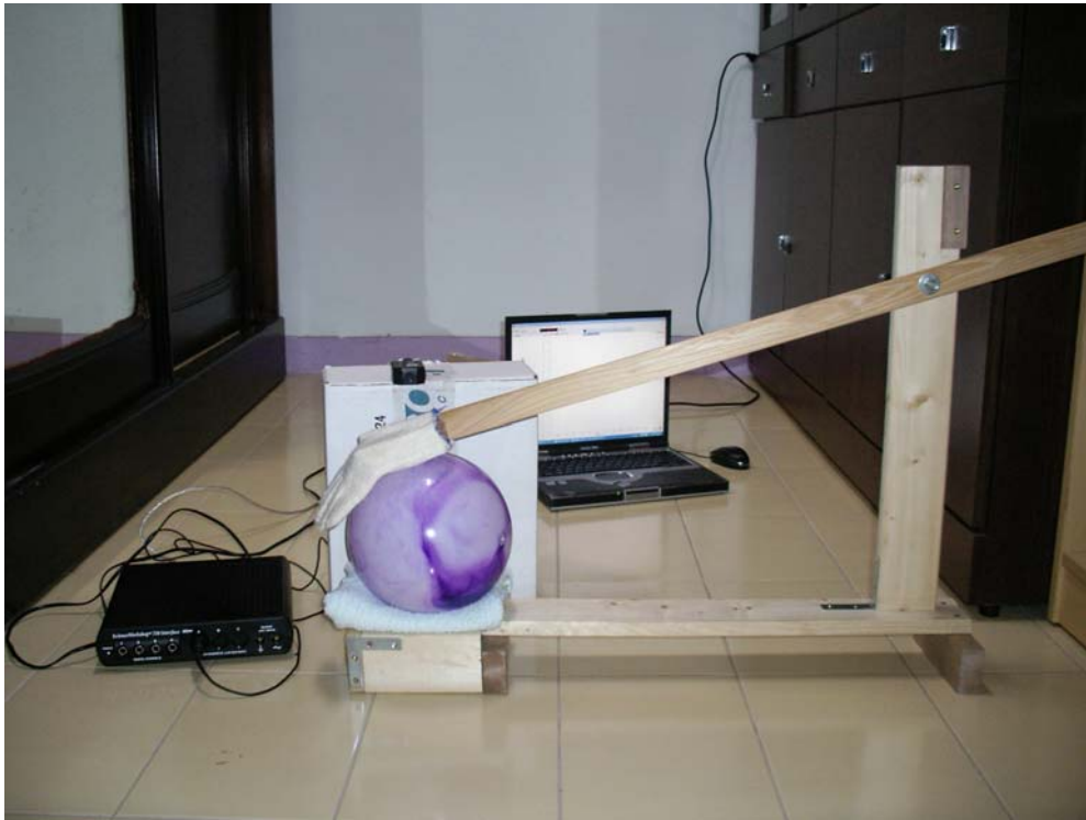
圖 1 拍擊裝置
