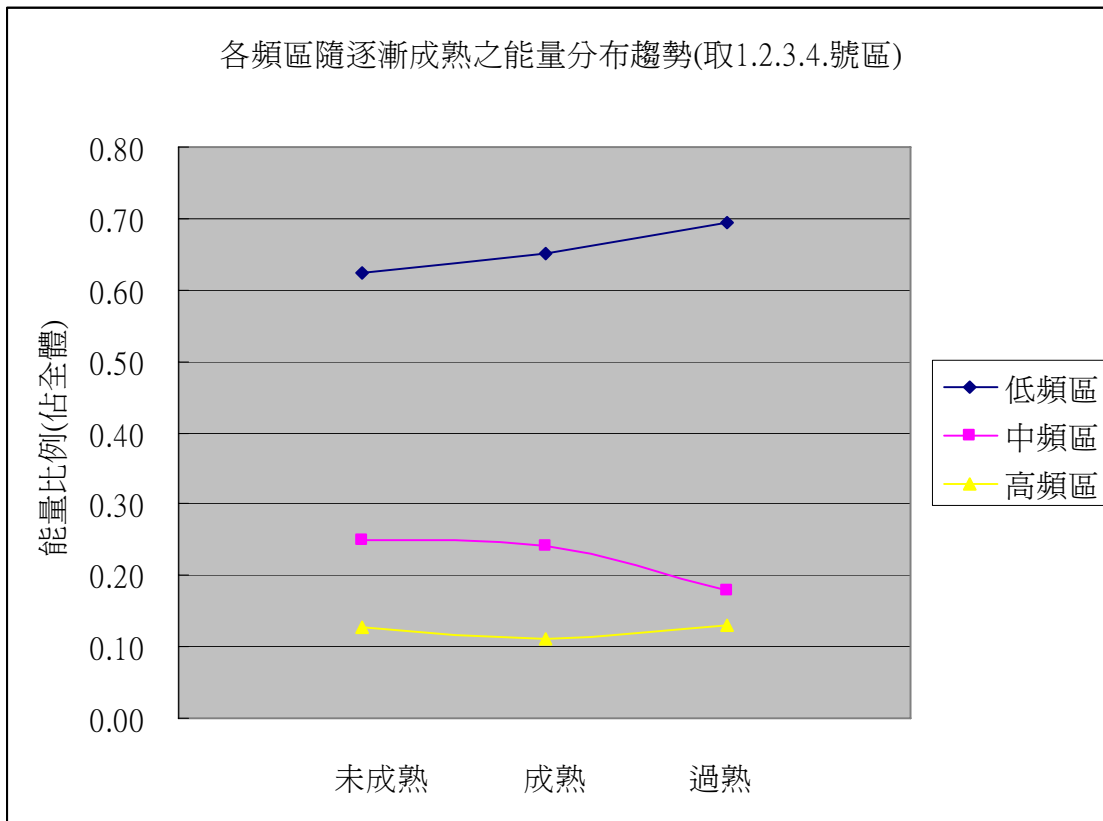
圖 16 隨成熟度之增加，各頻區之能量分佈變化圖（1-4 號拍擊點）
