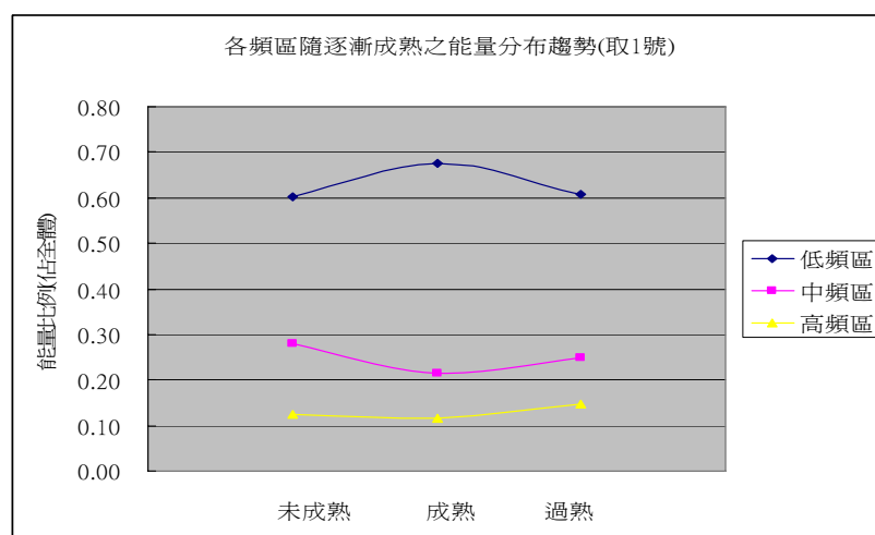
圖 11 隨成熟度之增加, 各頻區之能量分佈變化圖 (1 號拍擊點)
