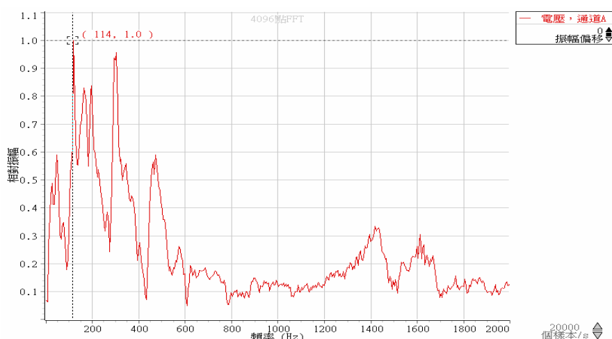
圖 21 未成熟西瓜一號拍擊點拍聲頻譜
