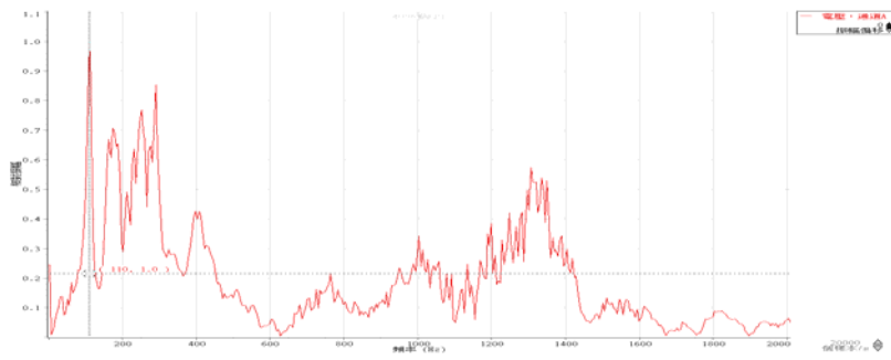
圖 22 同一顆未成熟西瓜二號拍擊點拍聲頻譜
