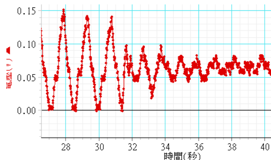
圖 (3-4) 港區內波浪衰退波形
