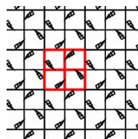
p4
