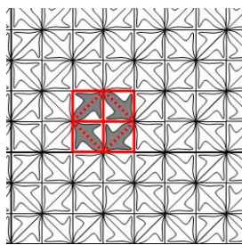
p4g
