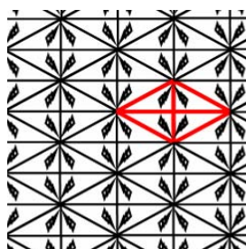
cmm
