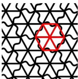
p6
