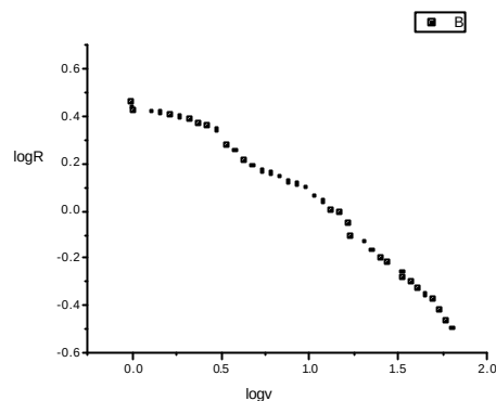
圖七：甘油的 \log R - \log v
