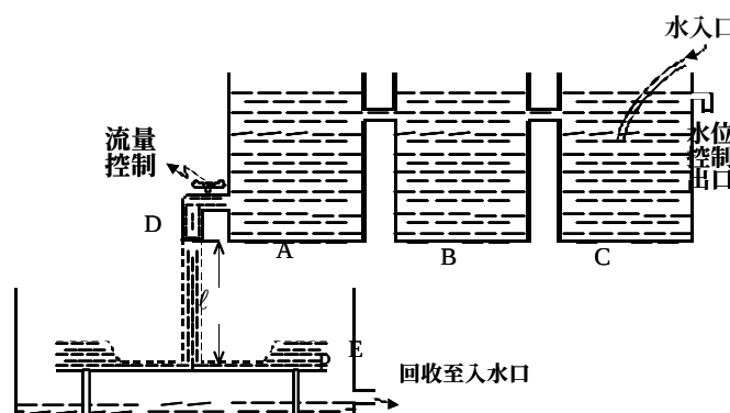
圖二：實驗裝置
