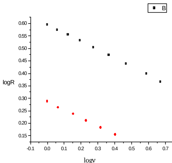
圖六：水(■)及酒精(●)之 \log R 對 \log v
