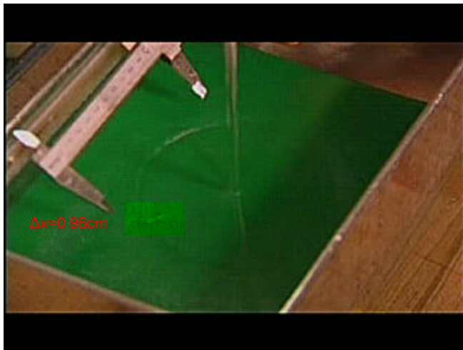
圖三(a) 碎片,在臨界點以內,1/30 秒移動 0.96cm,顯示出水的流速 29\text{cm/s} 。
