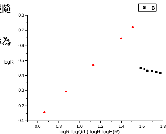
圖五：水的 \log R 對 \log Q 及 \log R 對 \log H 圖
