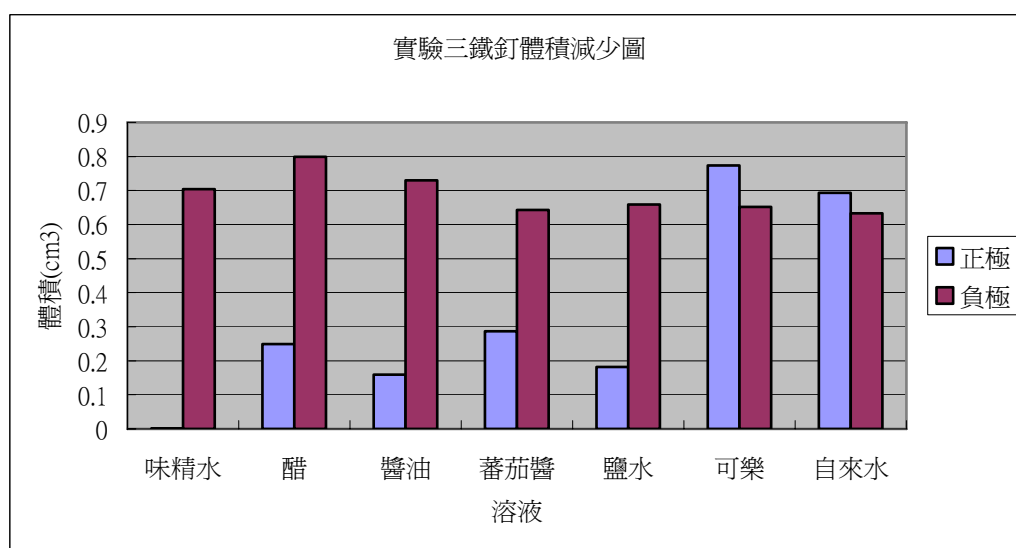
圖十二 實驗三：鐵釘體積減少圖
