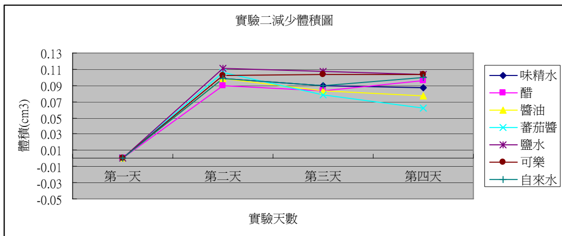
圖八 實驗二：金屬—不鏽鋼體積減少圖
