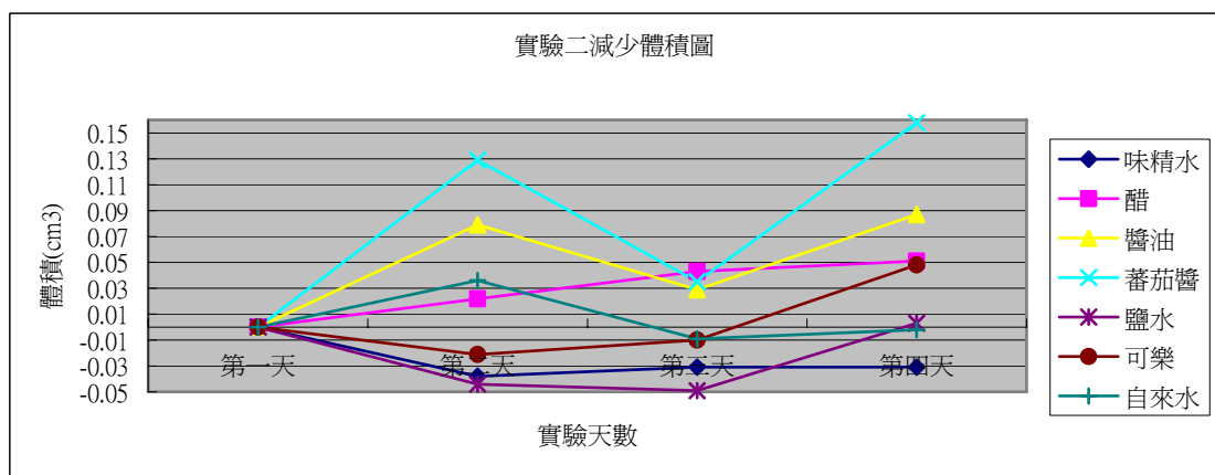
圖九 實驗二：金屬—鋁體積減少圖
