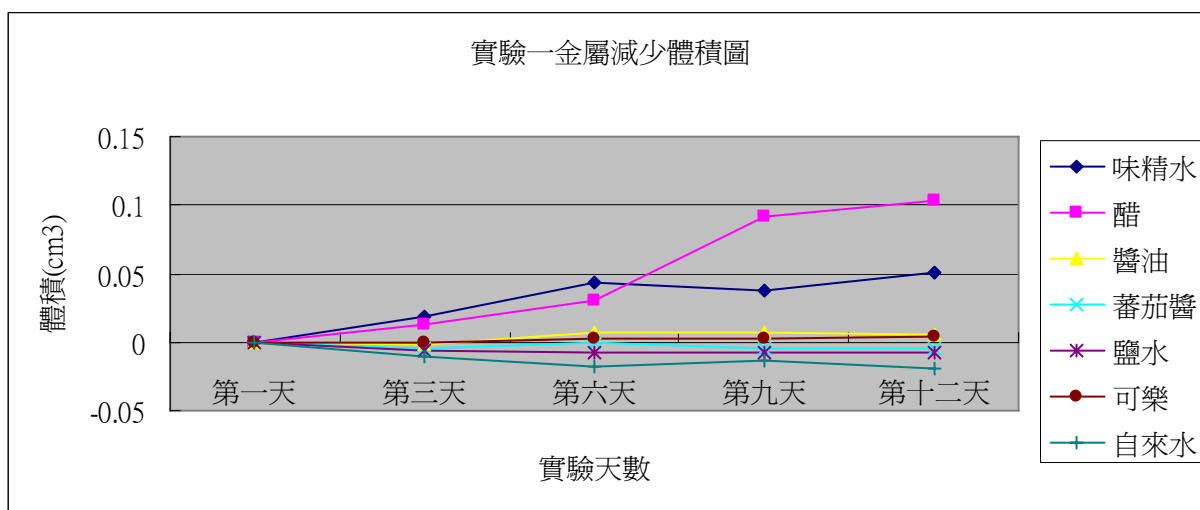
圖六 實驗一：金屬— 鋅 體積減少圖
