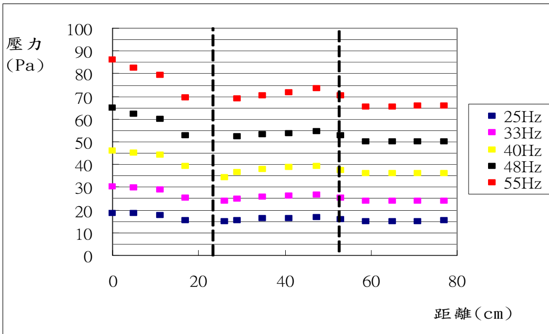
圖 2-2-7 紗網 C，各點的壓力分佈圖
