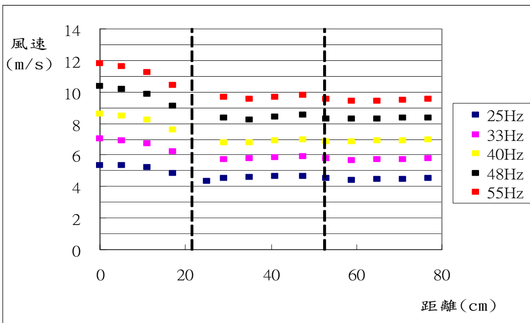
圖 2-2-4 紗網 B，各點的風速分佈圖
