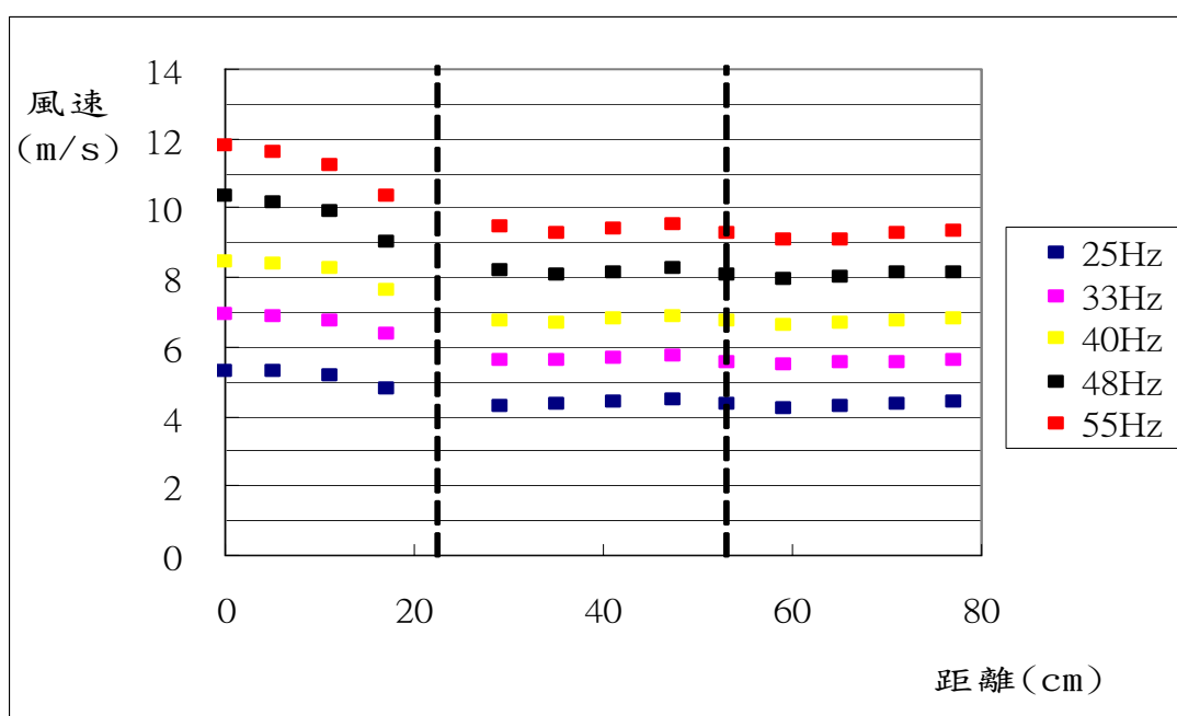
圖 2-2-2 紗網 A，各點的風速分佈圖
