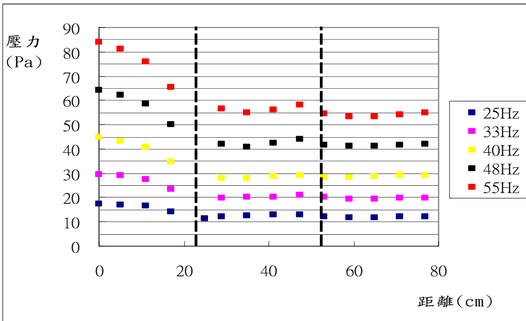
圖 2-2-5 紗網 B，各點的壓力分佈圖
