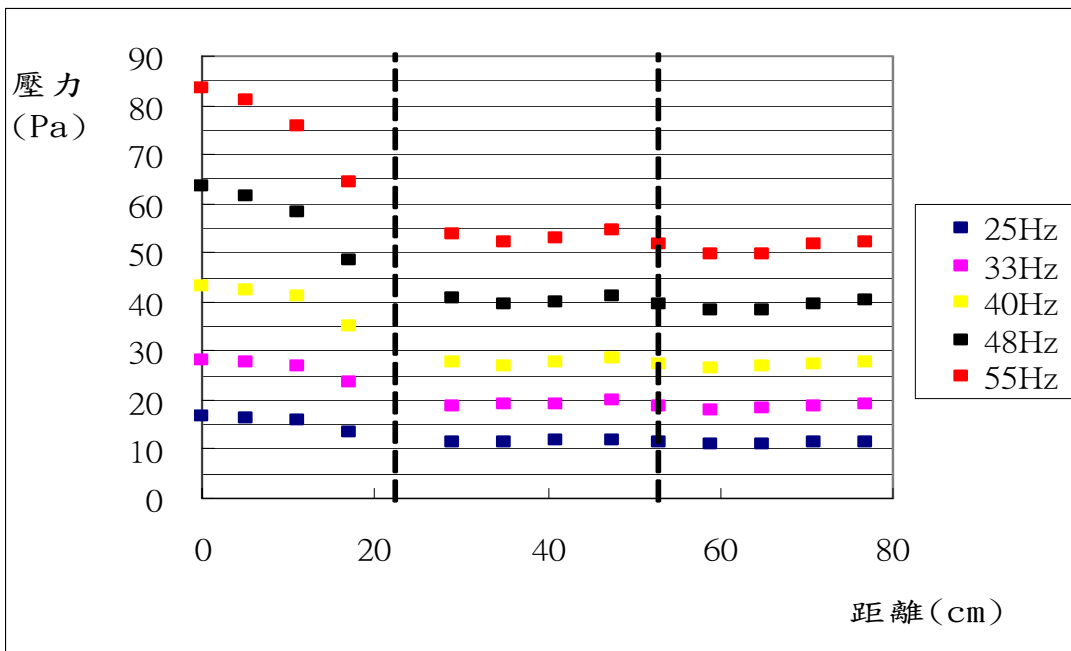
圖 2-2-3 紗網 A，各點的壓力分佈圖
