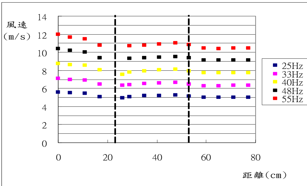
圖 2-2-6 紗網 C，各點的風速分佈圖
