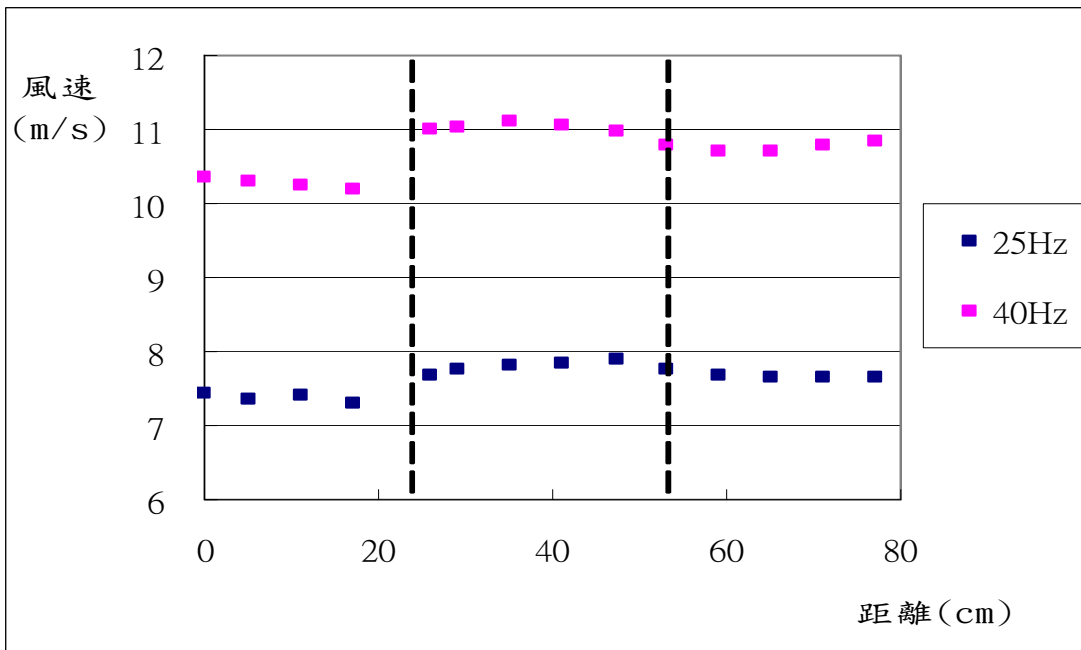
圖 2-2-8 紗網 D，各點的風速分佈圖
