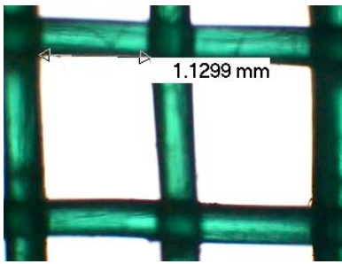
圖七 網徑 1.13mm
