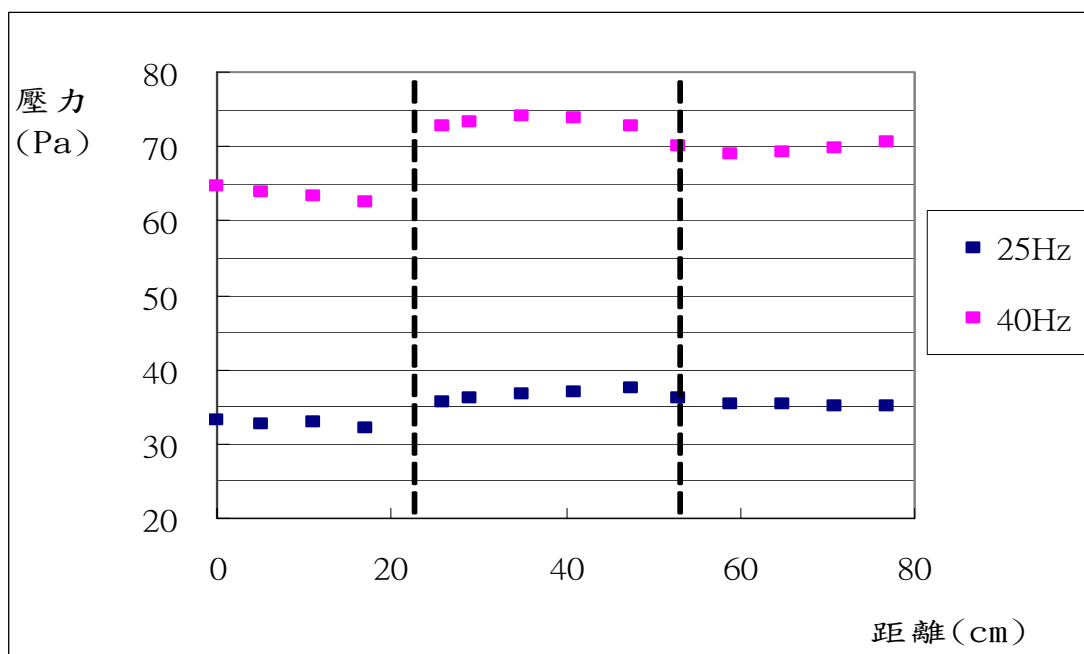
圖 2-2-9 紗網 D，各點的壓力分佈圖
