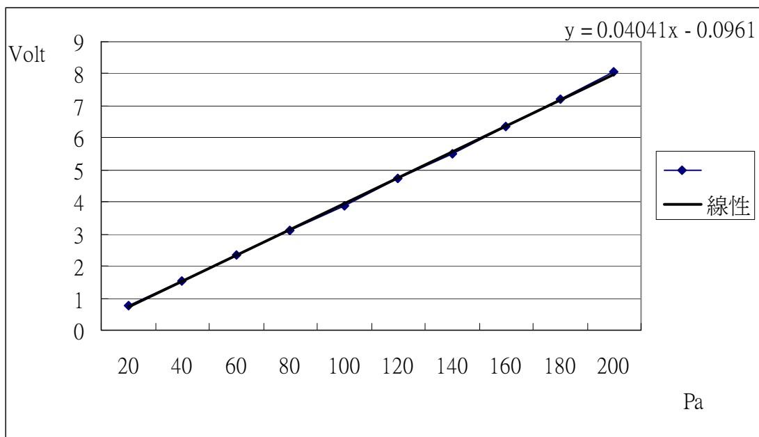
圖 2-1-1 Channel 1 校正曲線
