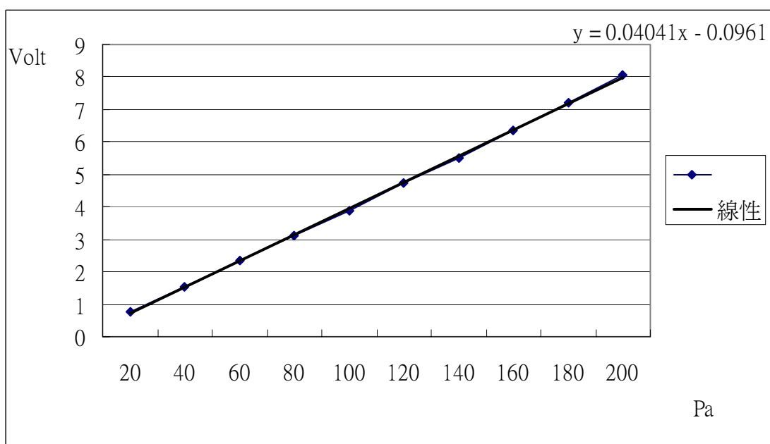
圖 2-1-2 Channel 2 校正曲線
