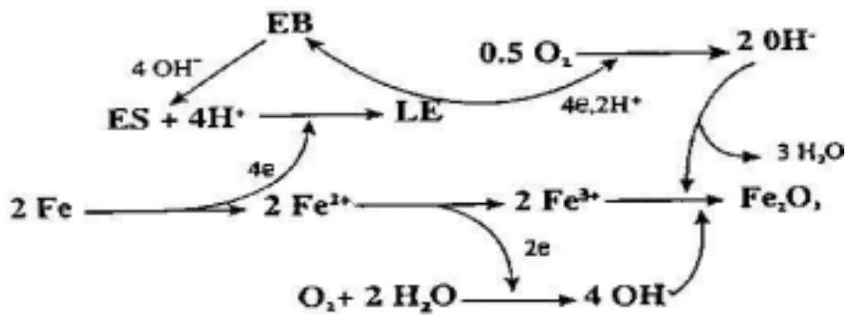
圖 1 聚苯胺防蝕反應機構
