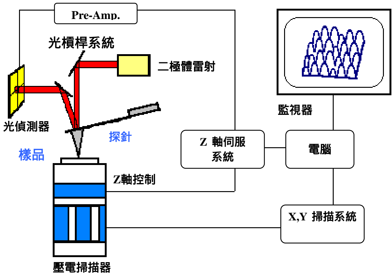
圖3 AFM的成像原理示意圖
