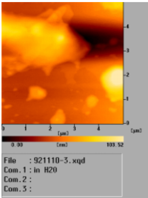
圖 7 以純化過的聚苯胺添加最佳比例之界面活性劑製備的聚苯胺 AFM 圖（未使用 HCl）
