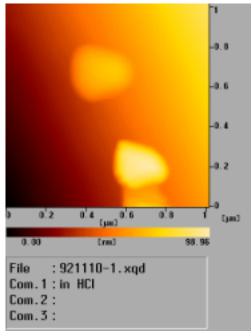
圖 8 以純化過的聚苯胺添加最佳比例之界面活性劑製備的聚苯胺 AFM 圖（使用 HCl）
