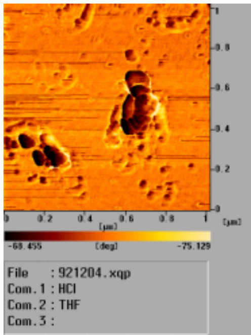
圖 9 以純化過的聚苯胺添加最佳比例之界面活性劑製備的聚苯胺 AFM 圖（以 THF 溶解聚苯胺粒子）
