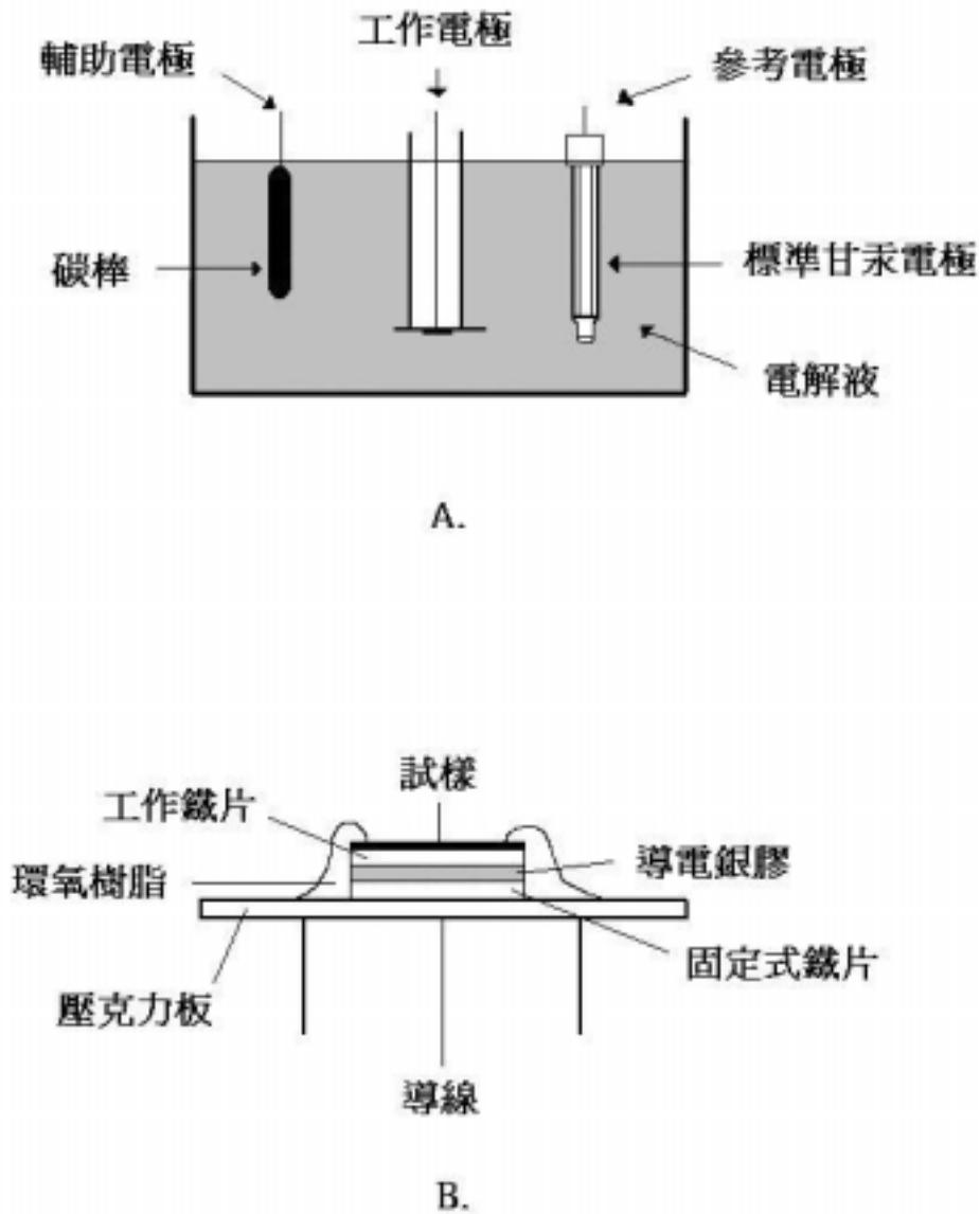
圖 4 A.循環伏特安培儀工作裝置圖；B.工作電極剖面圖
