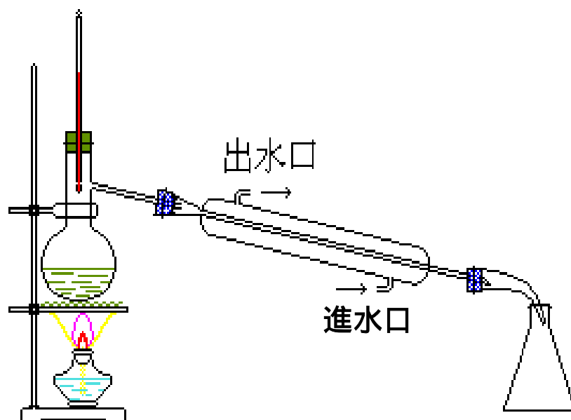
圖 2 純化苯胺單體裝置圖。
