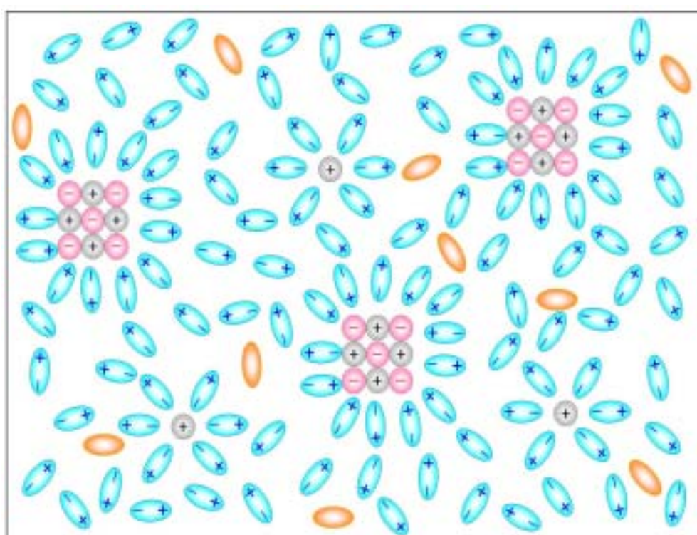
有添加物之離子晶體的酒精凝膠的分子模型圖
