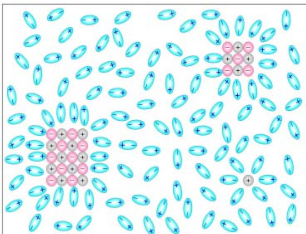
離子晶體的酒精凝膠開始溶出酒精的分子模型圖
