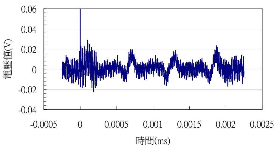
圖 6：線圈匝數為 125 匝的感應訊號。
