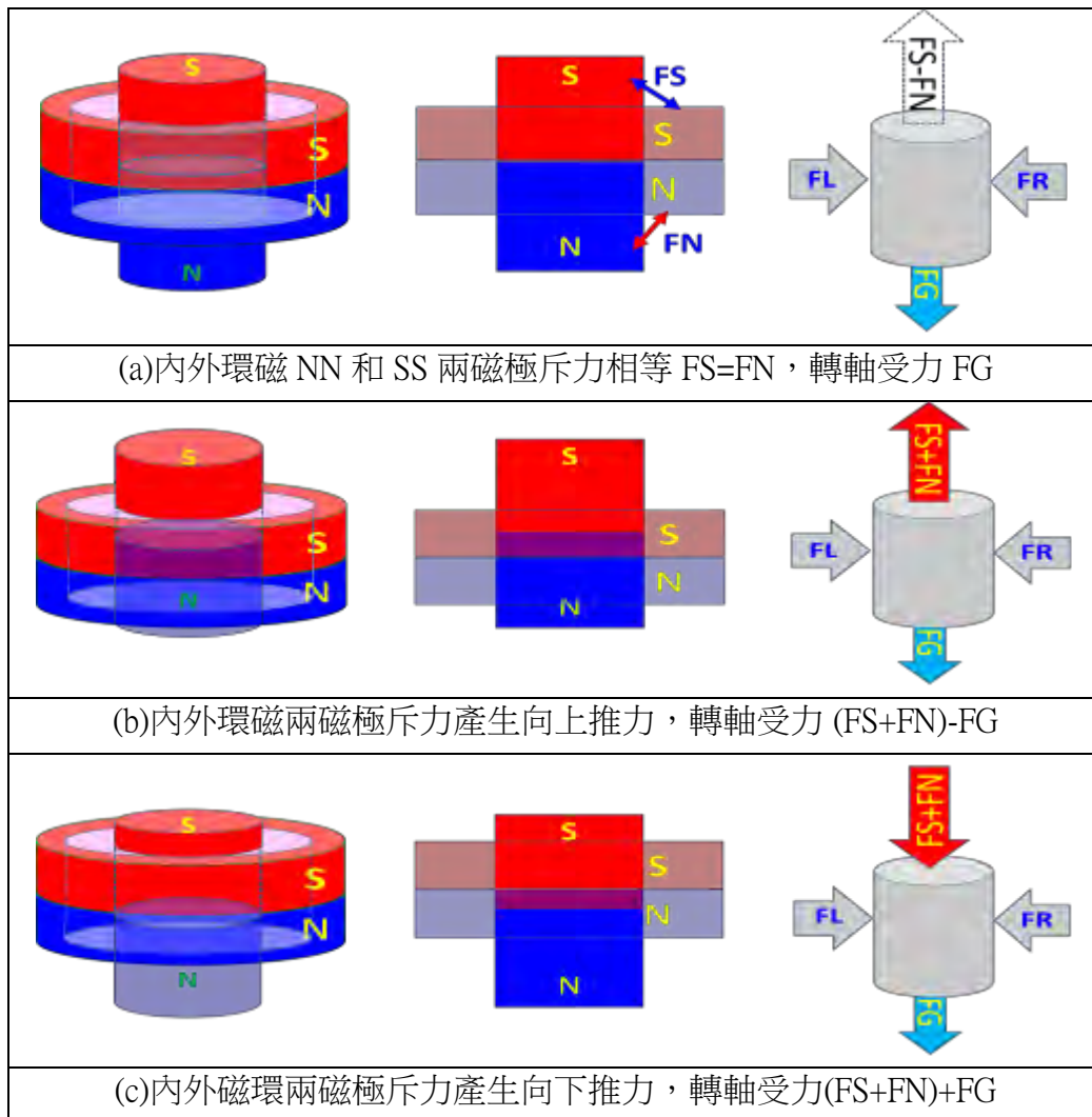
圖 20、內外環磁磁力作用與轉軸的受力分析圖示
