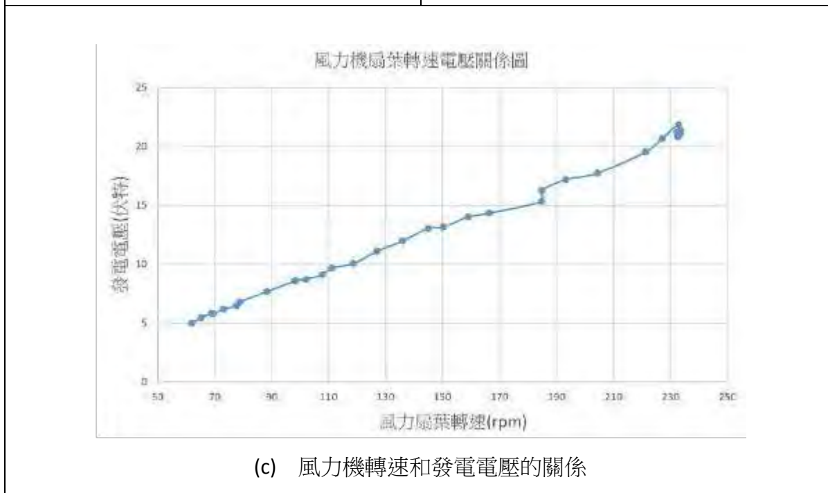
圖 25、風力機轉動效能分析
