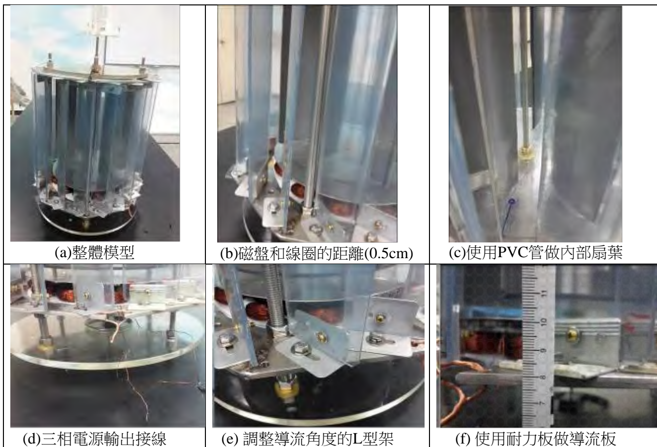
圖 24、風力機模型各部件特寫
