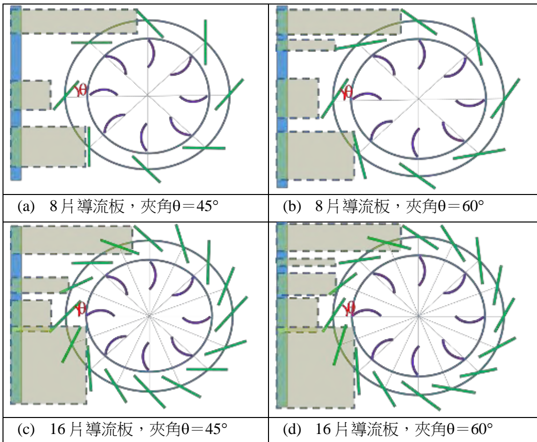
圖 16、導流板角度和數目對於風力的影響
