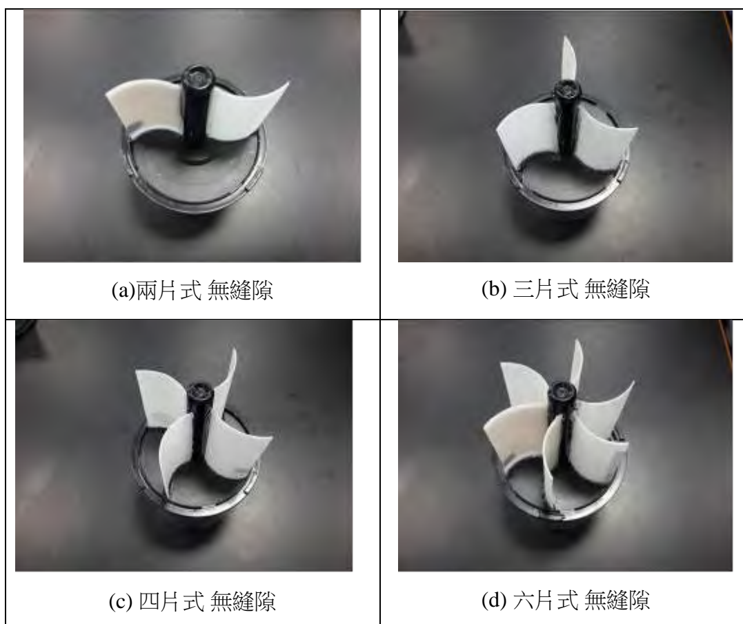
圖 2、無縫隙風力扇葉
