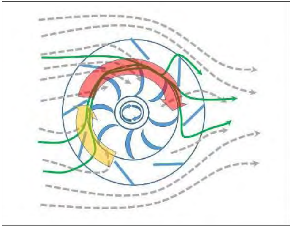
圖 11、起霧器觀察氣流現象，吹進來的右邊或左邊的風經導流之後都轉成順向力矩，右邊以黃色箭頭，左邊以紅色箭頭表示轉向。
